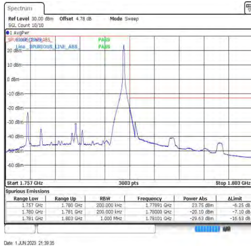
Band66-20MHz-QPSK-132572-1RB#99
