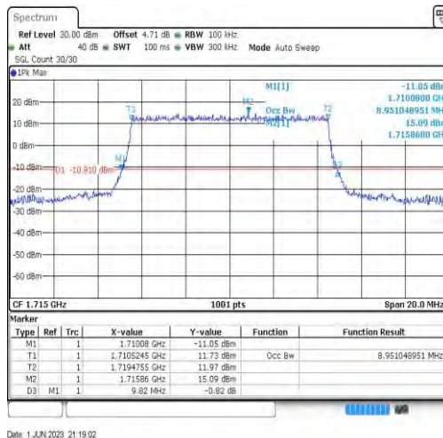
Band66-10MHz-QPSK-132022-50RB#0-8.951
