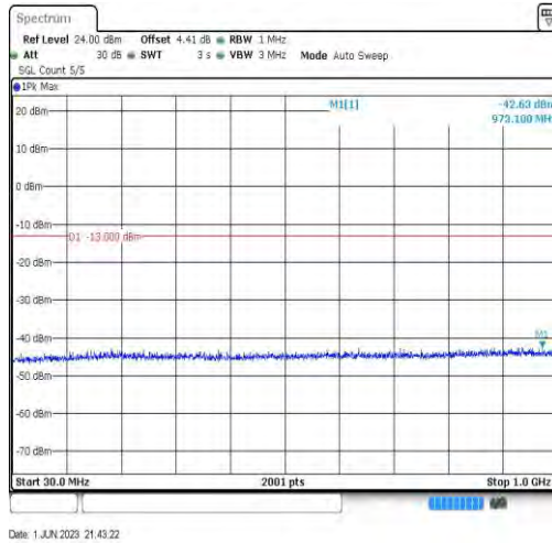
Band66-20MHz-QPSK-132572-1RB#0-Range3:30~1000MHz
