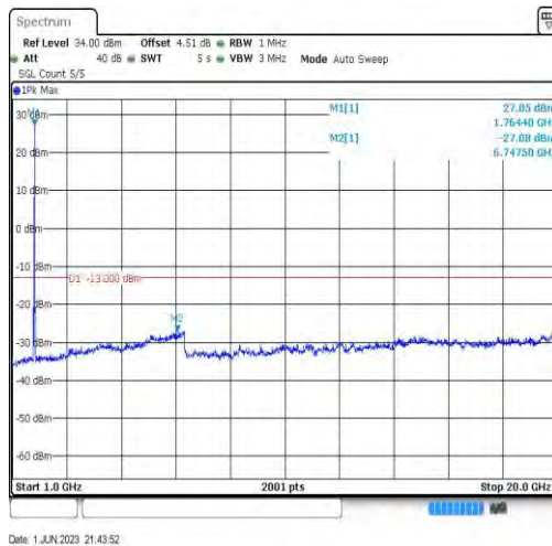
Band66-20MHz-QPSK-132572-1RB#0-Range4:1000~20000MHz
