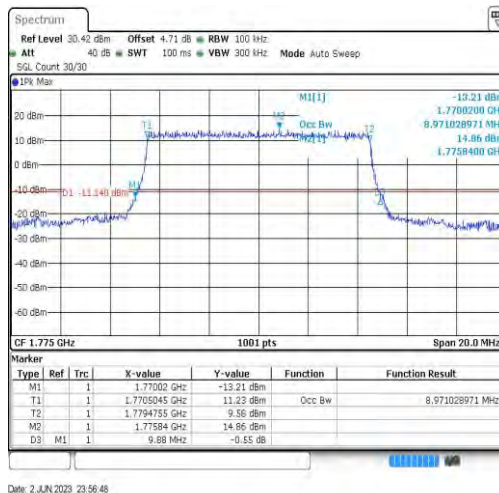
Band66-10MHz-QPSK-132622-50RB#0-8.971
