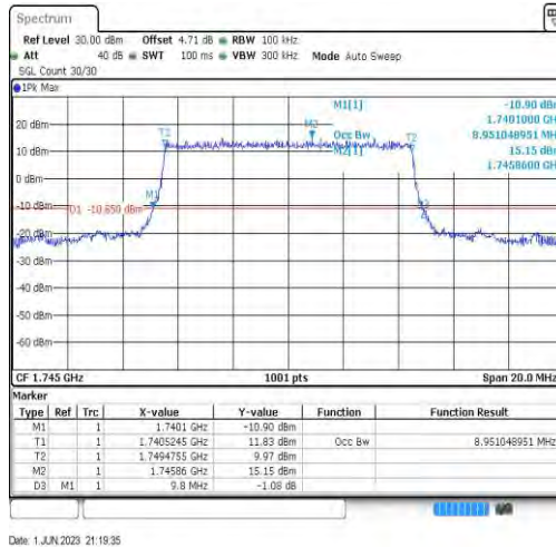
Band66-10MHz-QPSK-132322-50RB#0-8.951
