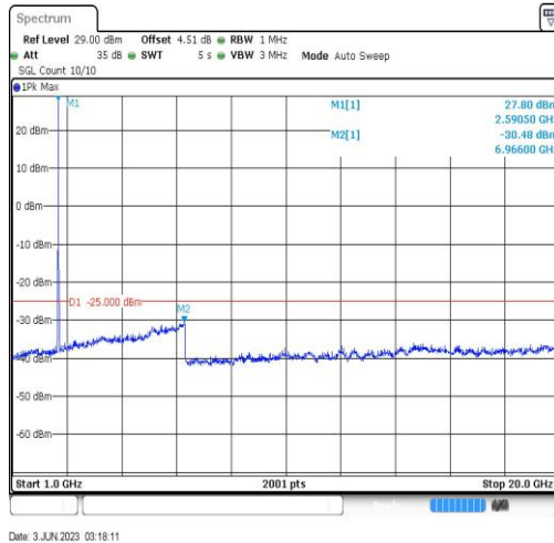
Band41-20MHz-QPSK-40640-1RB#0-Range4:1000~20000MHz
