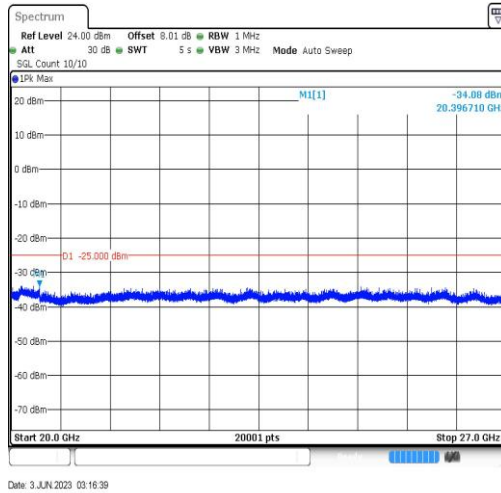
Band41-20MHz-QPSK-40140-1RB#0-Range5:20000~27000MHz
