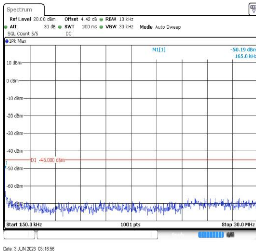
Band41-20MHz-QPSK-40640-1RB#0-Range2:0.15~30MHz
