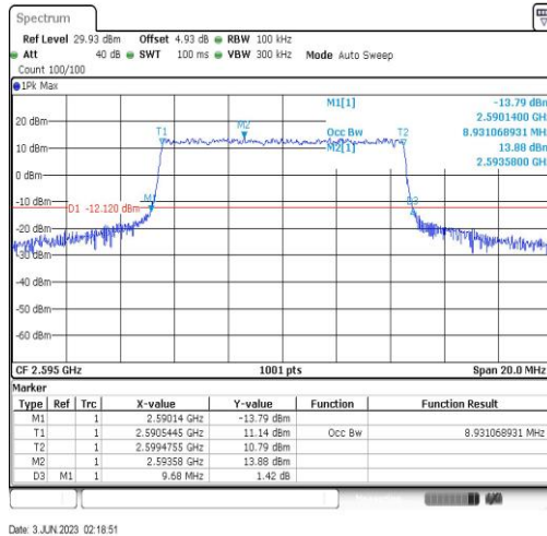
Band41-10MHz-QPSK-40640-50RB#0-8.931
