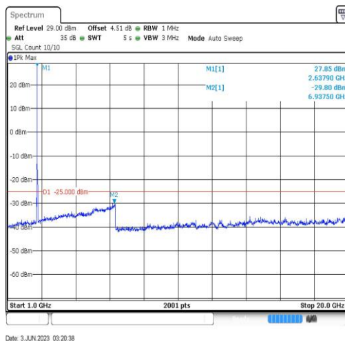
Band41-20MHz-QPSK-41140-1RB#0-Range4:1000~20000MHz
