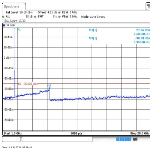
Band41-20MHz-QPSK-40140-1RB#0-Range4:1000~20000MHz
