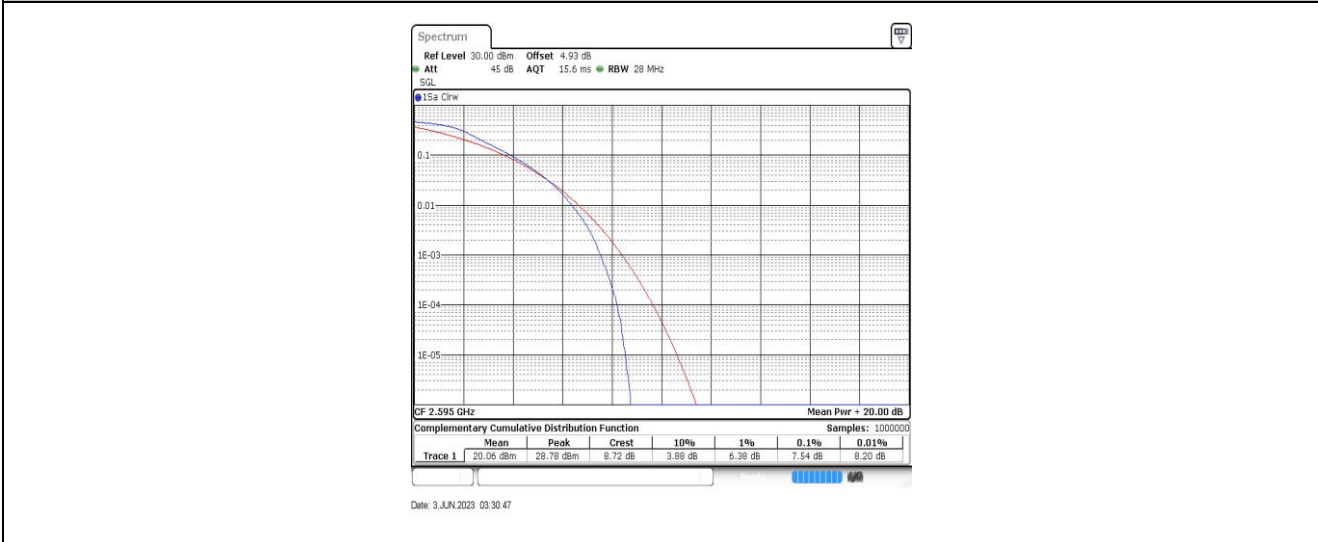
Band41-20MHz-QPSK-40640-100RB#0
