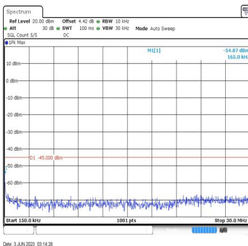
Band41-20MHz-QPSK-40140-1RB#0-Range2:0.15~30MHz
