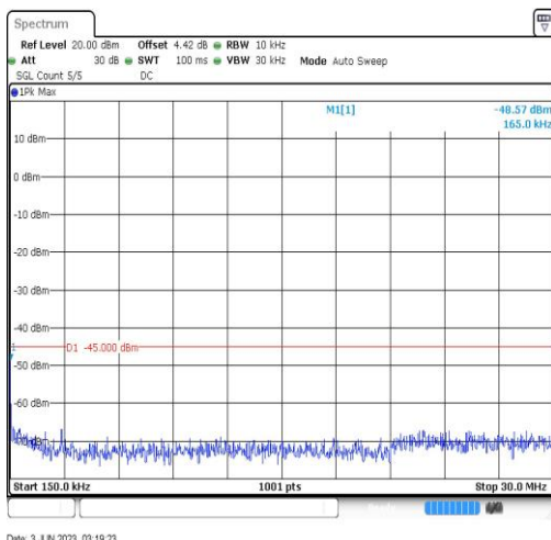
Band41-20MHz-QPSK-41140-1RB#0-Range2:0.15~30MHz
