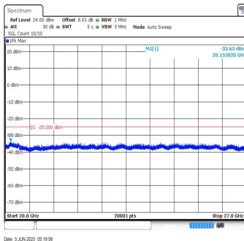
Band41-20MHz-QPSK-40640-1RB#0-Range5:20000~27000MHz
