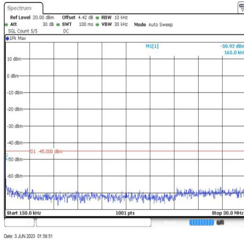
Band38-20MHz-QPSK-38000-1RB#0-Range2:0.15~30MHz
