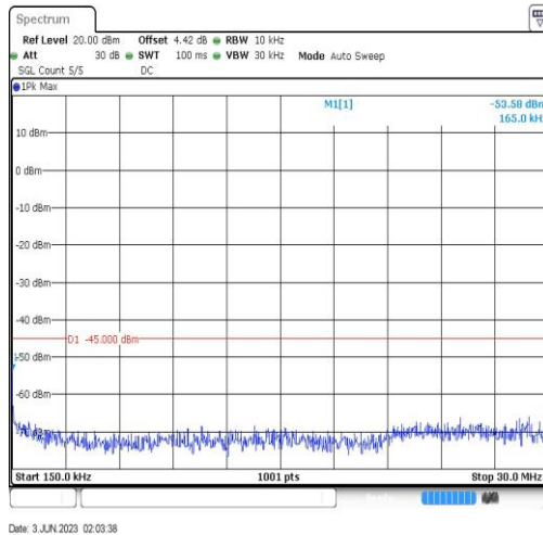
Band38-20MHz-QPSK-38150-1RB#0-Range2:0.15~30MHz
