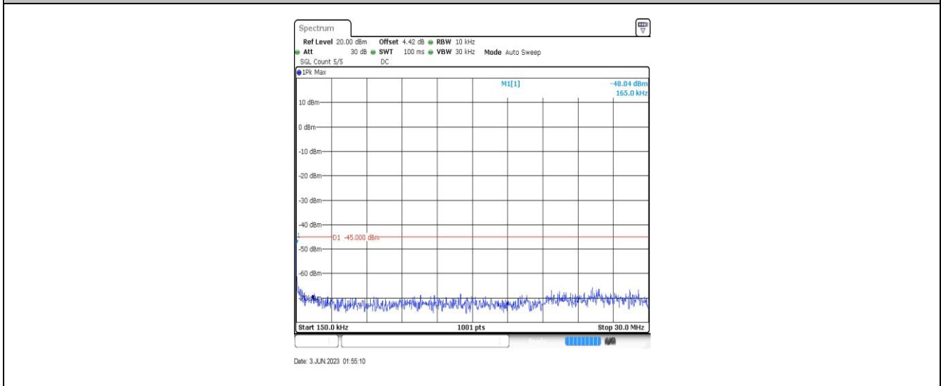
Band38-20MHz-QPSK-37850-1RB#0-Range2:0.15~30MHz
