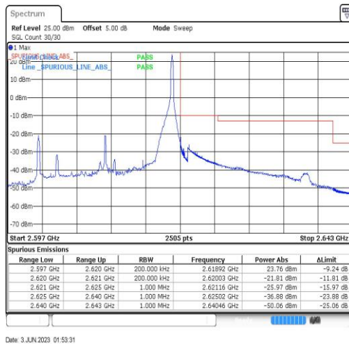
Band38-20MHz-QPSK-38150-1RB#99
