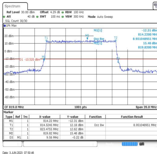
Band26-10MHz-QPSK-26740-50RB#0-8.951
