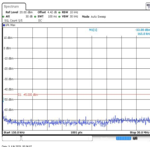
Band7-20MHz-QPSK-21350-1RB#0-Range2:0.15~30MHz
