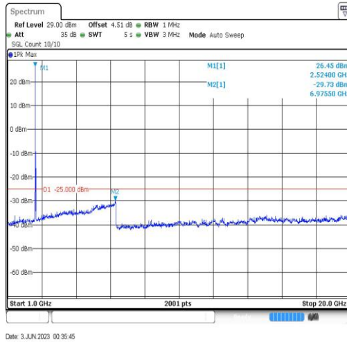
Band7-20MHz-QPSK-21100-1RB#0-Range4:1000~20000MHz
