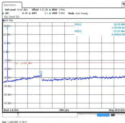
Band4-20MHz-QPSK-20050-1RB#0-Range4:1000~20000MHz
