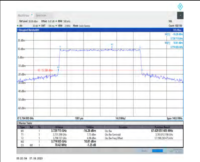
1-N78-3700-3800-PC3-30-70-H-8-CP-64QAM-Outer _Full-189@0-Ant1-67.429-70.420-≤70-PASS
