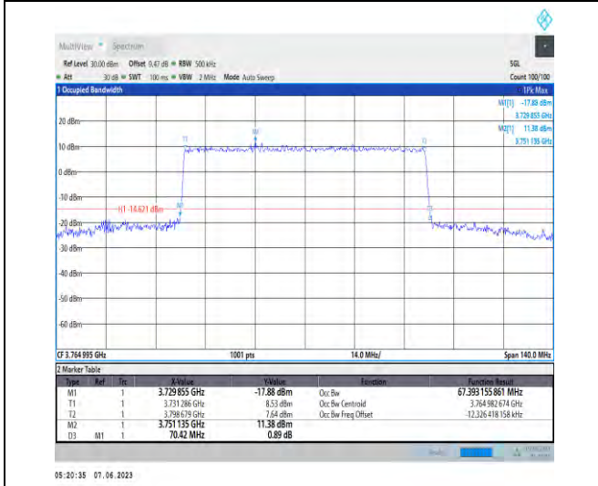
1-N78-3700-3800-PC3-30-70-H-7-CP-16QAM-Outer _Full-189@0-Ant1-67.393-70.420-≤70-PASS
