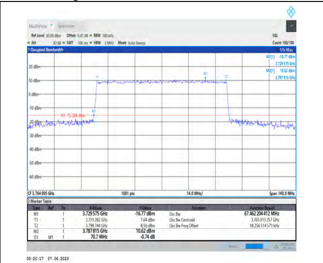
1-N78-3700-3800-PC3-30-70-H-6-CP-QPSK-Outer Full-189@0-Ant1-67.462-70.700-≤70-PASS
