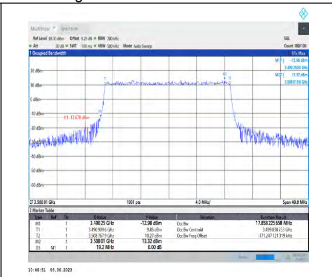
1-N78-3450-3550-PC3-30-20-M-3-DFT-16QAM-Outer_Full-50@0-Ant1-17.858-19.200-≤20-PASS
