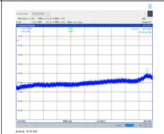
1-N78-3700-3800-PC3-30-100-M-1-N/A-DFT-PI2BPS K-Inner_1RB_Left-1@1-18000-40000-Ant1-18000.00 --62.35--13-PASS
