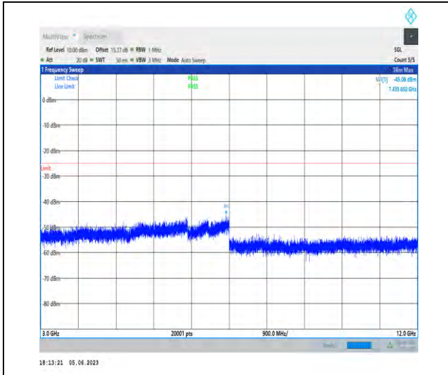
1-N41-PC3-30-100-L-1-N/A-DFT-PI2BPSK-Inner_1 RB_Left-1@1-3000-12000-Ant1-7435.65--45.08--25 -PASS
