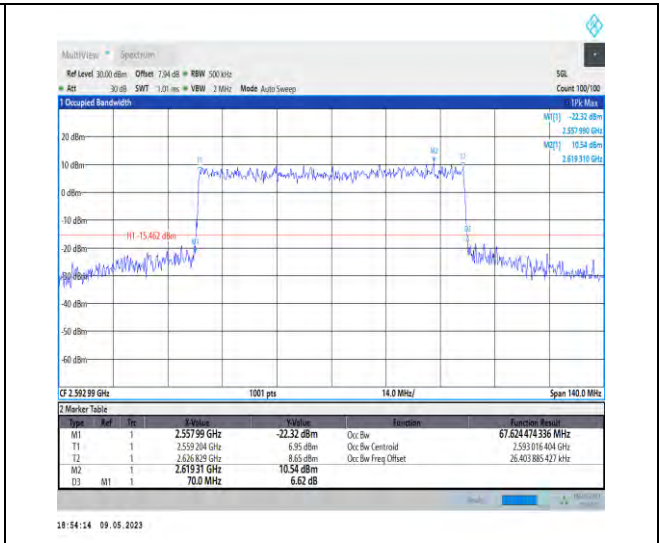
1-N41-PC3-30-70-M-8-CP-64QAM-Outer_Full-189 @0-Ant1-67.624-70.000-≤70-PASS
