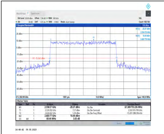
1-N41-PC3-30-70-M-7-CP-16QAM-Outer_Full-189@ 0-Ant1-67.37-69.440-≤70-PASS
