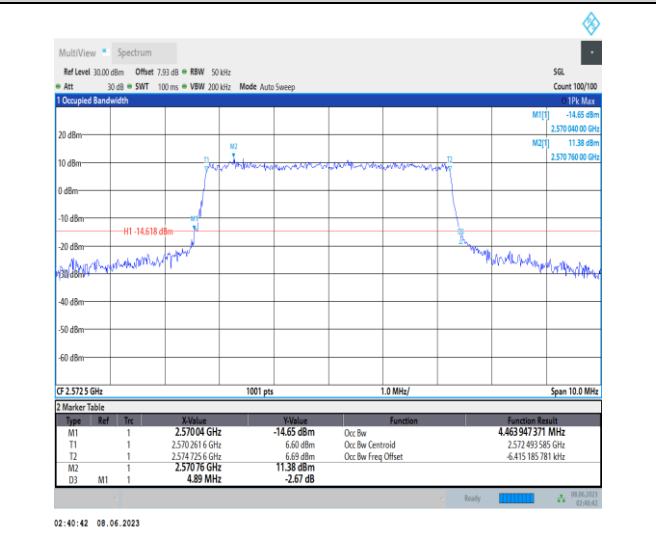
1-N38-PC3-15-5-L-8-CP-64QAM-Outer_Full-25@0-A nt1-4.464-4.890-≤5-PASS
