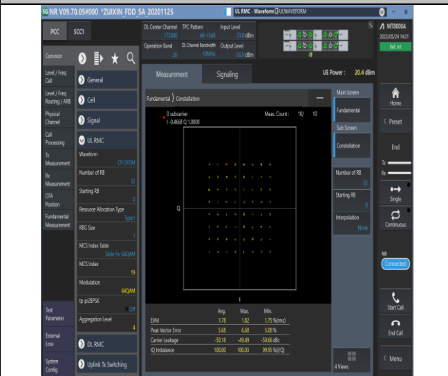
NTVN,N26-814-824,_PC3,_15,10,M,TID8,#1
