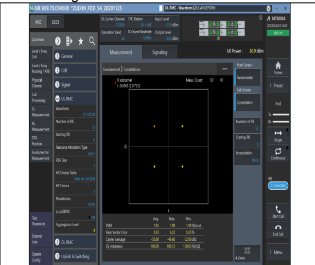
NTVN,N26-814-824,_PC3,_15,10,M,TID6,#1
