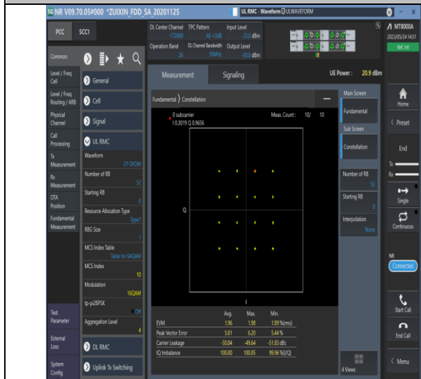
NTVN,N26-814-824,_PC3,_15,10,M,TID7,#1
