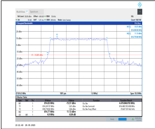
NTNV_N26-814-824_PC3_15_5_L_TID6_Ant1#1
