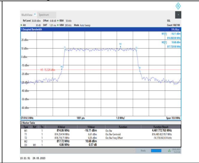
NTNV_N26-814-824_PC3_15_5_L_TID7_Ant1#1
