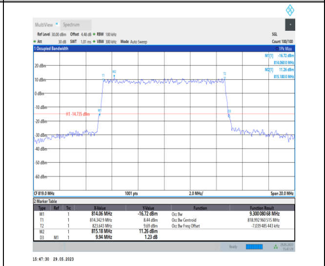
NTVN_N26-814-824_PC3_15_10_M_TID7_Ant1#1
