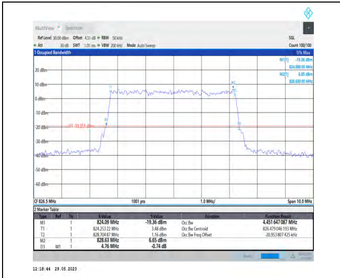
1-N5-PC3-15-5-L-9-CP-256QAM-Outer_Full-25@0-A nt1-4.452-4.760-≤5-PASS
