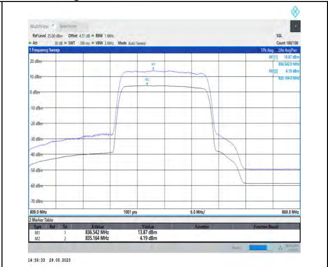
1-N5-PC3-15-20-H-2-CP-256QAM-Outer_Full-106@ 0-Ant1-9.68-100%-0.00-9.68-PASS-≤13
