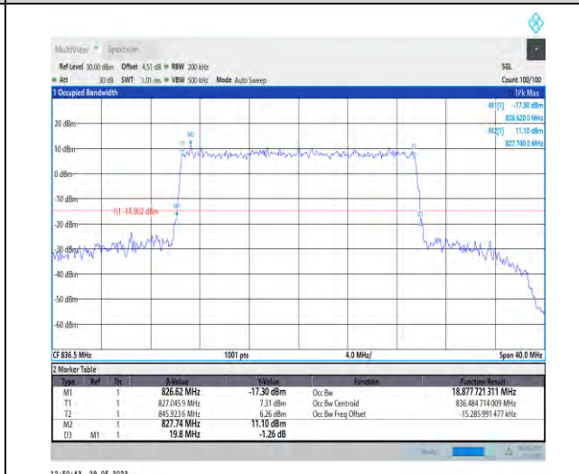
1-N5-PC3-15-20-M-8-CP-64QAM-Outer_Full-106@ 0-Ant1-18.878-19.800-≤20-PASS
