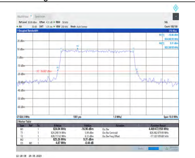
1-N5-PC3-15-5-L-6-CP-QPSK-Outer_Full-25@0-Ant 1-4.469-4.870-≤5-PASS
