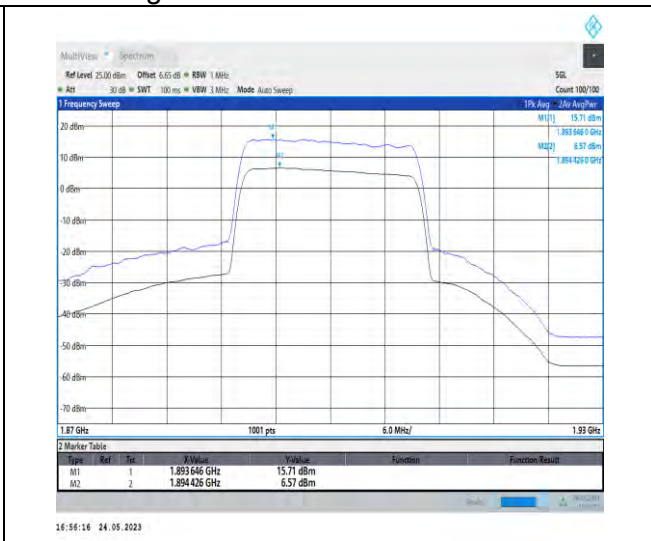
1-N2-PC3-15-20-H-2-CP-256QAM-Outer_Full-106@ 0-Ant1-9.14-100%-0.00-9.14-PASS-≤13
