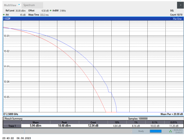
38-38-20MHz-20MHz-QPSK-QPSK-37901-38099-100RB#0-100RB#0
