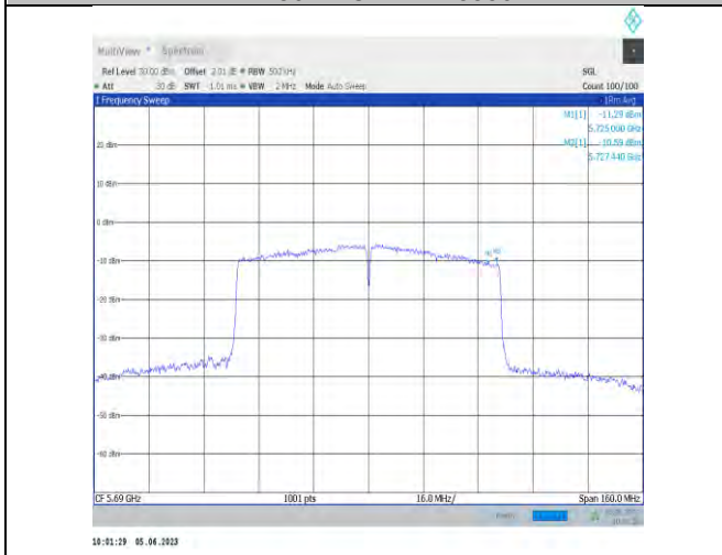
11ac80SISO-Ant22-5690 UNII-3
