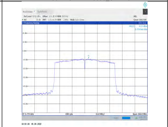
11ac80SISO-Ant22-5775
