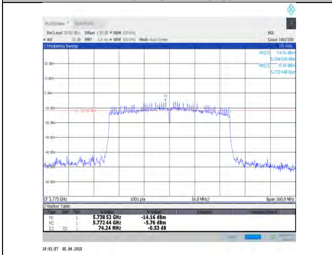
11ac80SISO-Ant22-5775
