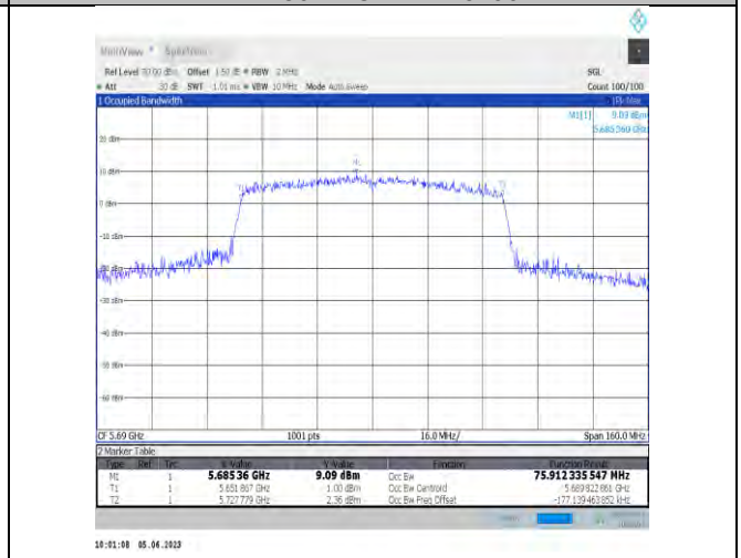
11ac80SISO-Ant22-5690
