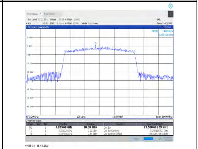
11ac80SISO-Ant22-5290
