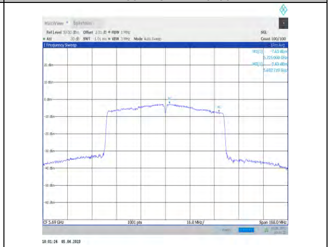
11ac80SISO-Ant22-5690 UNII-2C
