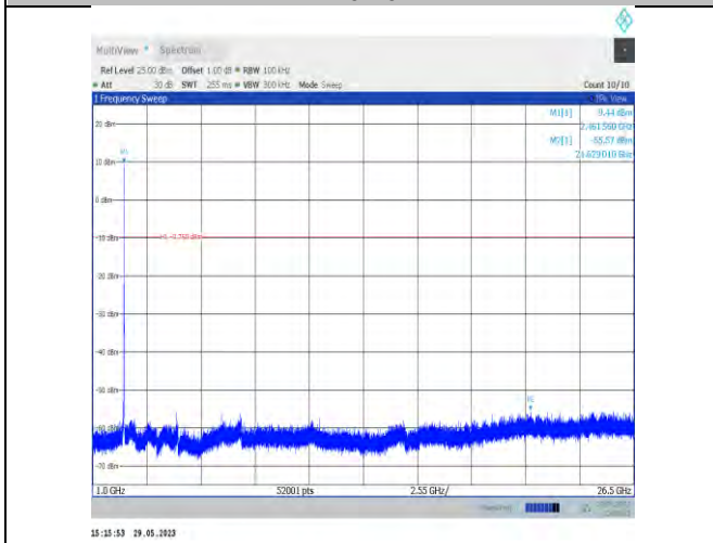
11b-Ant22-2462-1000~26500
