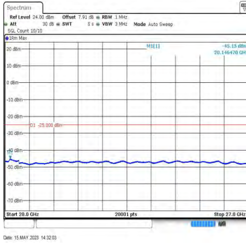
41-41-20MHz-20MHz-QPSK-QPSK-41292-41490-1RB#0-0RB#0-20000~27000MHz
