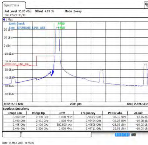
41-41-10MHz-20MHz-QPSK-QPSK-39705-39849-1RB#0-0RB#0
