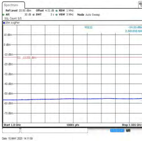
41-41-20MHz-20MHz-QPSK-QPSK-41292-41490-1RB#0-0RB#0-1000~2505MHz
