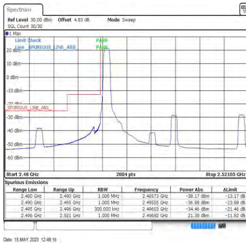
41-41-5MHz-20MHz-QPSK-QPSK-39683-39800-1RB#0-0RB#0
