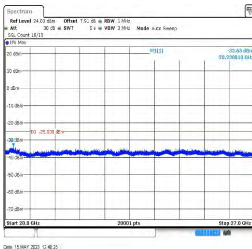
7-7-20MHz-20MHz-QPSK-QPSK-21001-21199-1RB#0-0RB#0-20000~27000MHz
