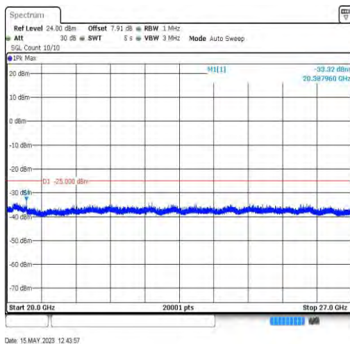
7-7-20MHz-20MHz-QPSK-QPSK-21152-21350-1RB#0-0RB#0-20000~27000MHz
