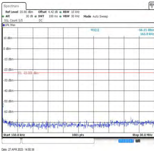
Band66-20MHz-QPSK-132572-1RB#0-Range2:0.15~30MHz
