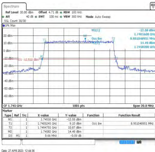
Band66-10MHz-QPSK-132322-50RB#0-8.951
