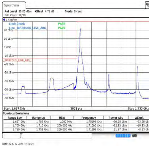
Band66-20MHz-QPSK-132072-1RB#0
