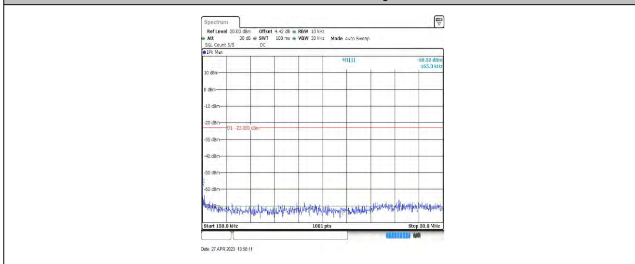
Band66-20MHz-QPSK-132072-1RB#0-Range2:0.15~30MHz
