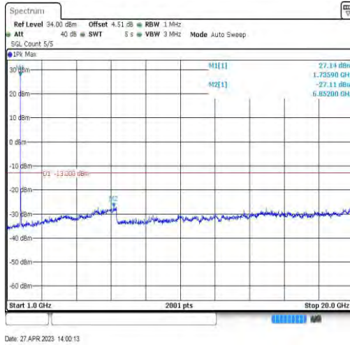
Band66-20MHz-QPSK-132322-1RB#0-Range4:1000~20000MHz
