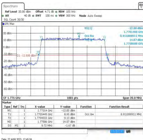
Band66-10MHz-QPSK-132622-50RB#0-8.911
