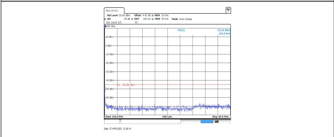
Band41-20MHz-QPSK-39750-1RB#0-Range2:0.15~30MHz
