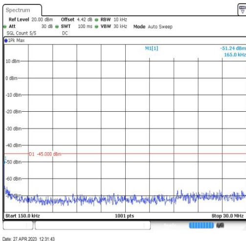
Band41-20MHz-QPSK-40620-1RB#0-Range2:0.15~30MHz
