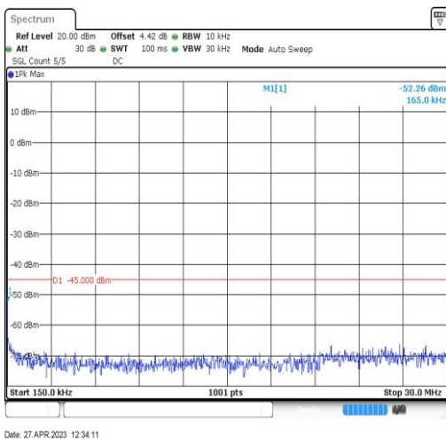
Band41-20MHz-QPSK-41490-1RB#0-Range2:0.15~30MHz
