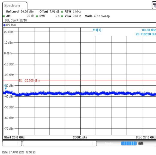
Band41-20MHz-QPSK-41490-1RB#0-Range5:20000~27000MHz
