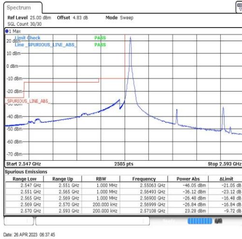
Band38-20MHz-QPSK-37850-1RB#0
