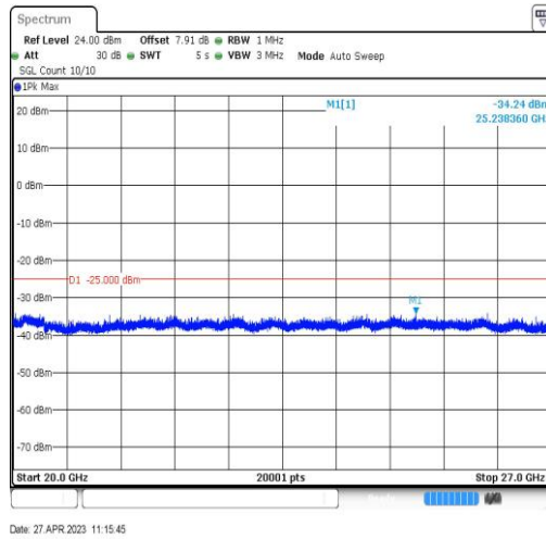
Band38-20MHz-QPSK-38150-1RB#0-Range5:20000~27000MHz
