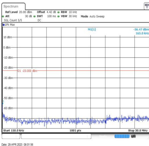
Band17-10MHz-QPSK-23800-1RB#0-Range2:0.15~30MHz
