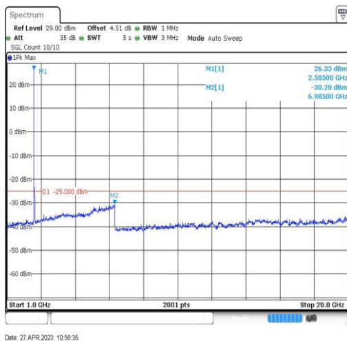
Band7-20MHz-QPSK-20850-1RB#0-Range4:1000~20000MHz
