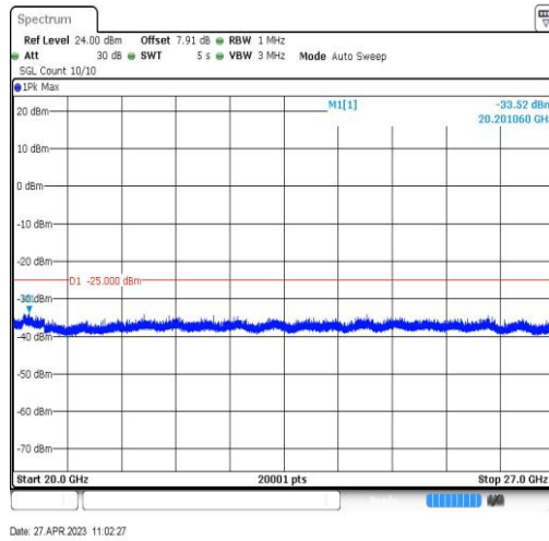
Band7-20MHz-QPSK-21350-1RB#0-Range5:20000~27000MHz
