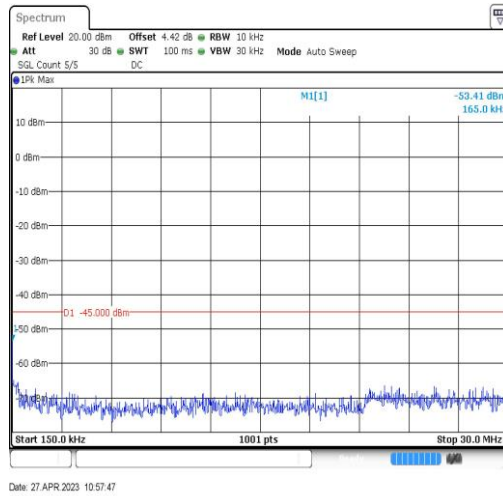
Band7-20MHz-QPSK-21100-1RB#0-Range2:0.15~30MHz
