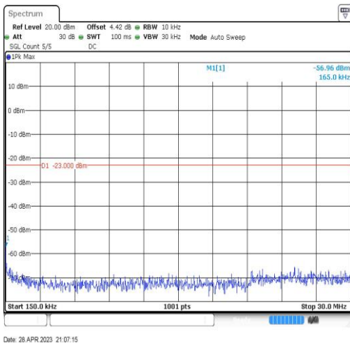
Band5-10MHz-QPSK-20525-1RB#0-Range2:0.15~30MHz
