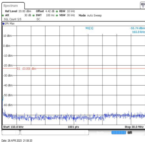
Band5-10MHz-QPSK-20600-1RB#0-Range2:0.15~30MHz
