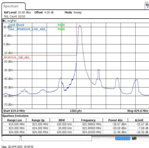
Band5-3MHz-QPSK-20415-1RB#0
