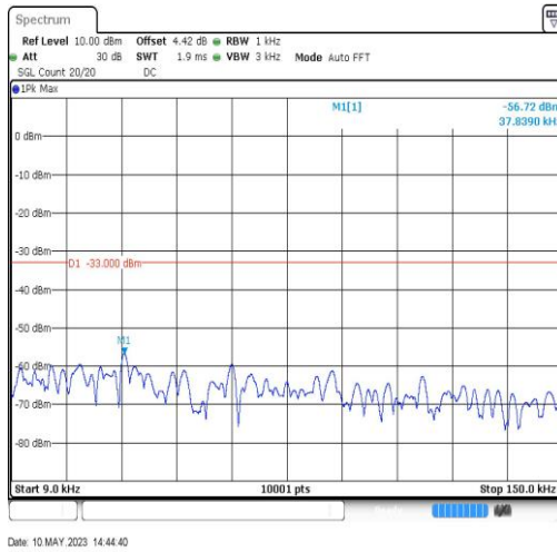
EGPRS850-251-8-0.009~0.15MHz-0.04
