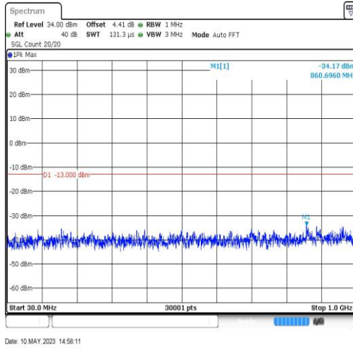
EGPRS1900-512-2-30~1000MHz-860.7
