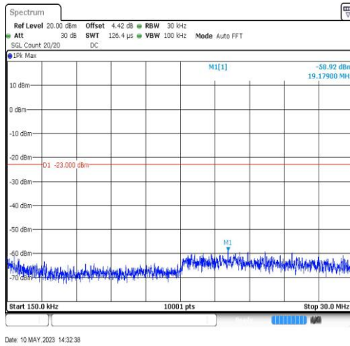
GSM1900-810-0-0.15~30MHz-19.18
