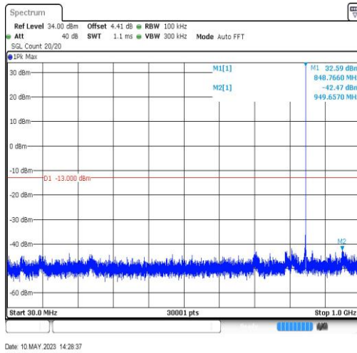
GSM850-128-5-30~1000MHz-949.66
