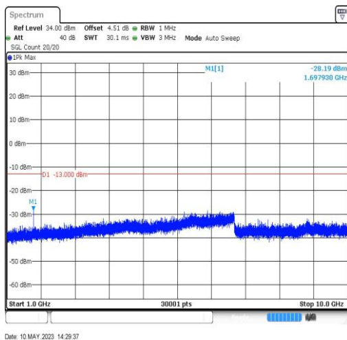
GSM850-251-5-1000~10000MHz-1697.93
