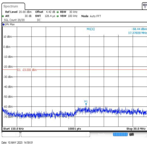
EGPRS1900-810-2-0.15~30MHz-17.37
