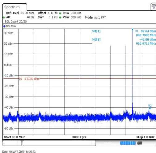
GSM850-251-5-30~1000MHz-959.97
