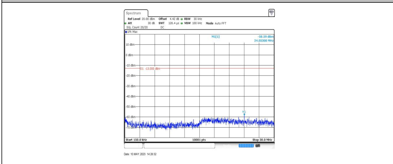
GSM850-128-5-0.15~30MHz-24.05
