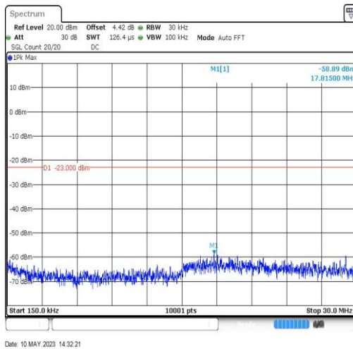
GSM1900-661-0-0.15~30MHz-17.82
