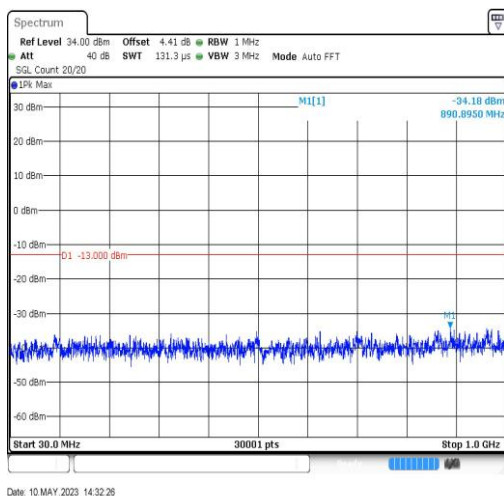
GSM1900-661-0-30~1000MHz-890.9
