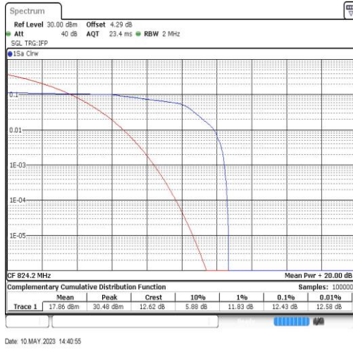
EGPRS850-128-8
