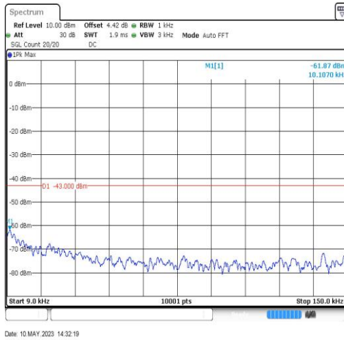
GSM1900-661-0-0.009~0.15MHz-0.01
