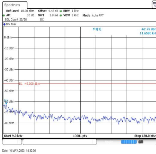
GSM1900-810-0-0.009~0.15MHz-0.01
