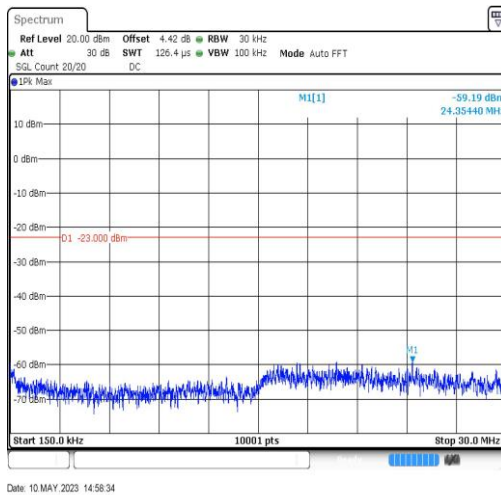
EGPRS1900-661-2-0.15~30MHz-24.35
