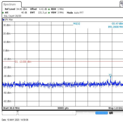
EGPRS1900-810-2-30~1000MHz-891.28
