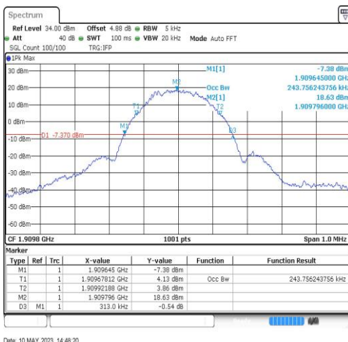
EGPRS1900-810-2
