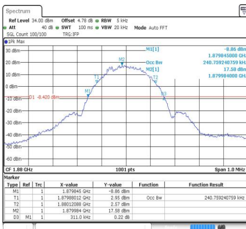
EGPRS1900-661-2
