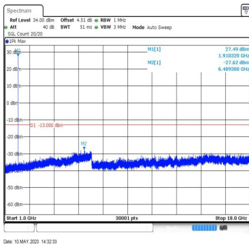
GSM1900-661-0-1000~18000MHz-6489.3
