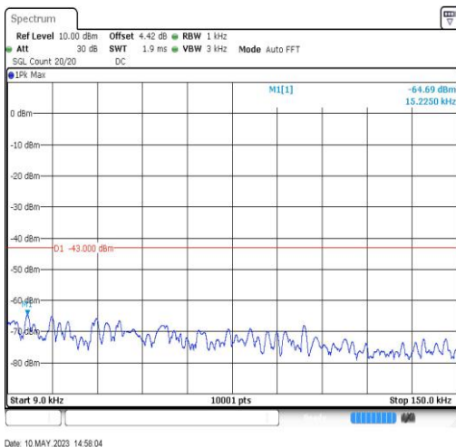
EGPRS1900-512-2-0.009~0.15MHz-0.02
