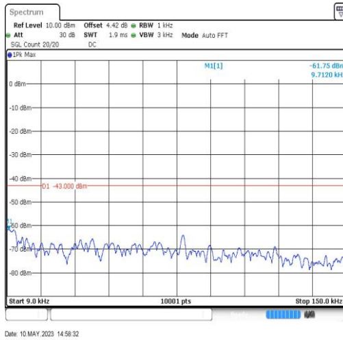
EGPRS1900-661-2-0.009~0.15MHz-0.01
