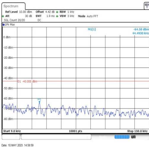
EGPRS1900-810-2-0.009~0.15MHz-0.04
