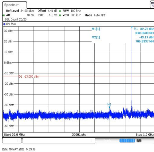
GSM850-190-5-30~1000MHz-706.83
