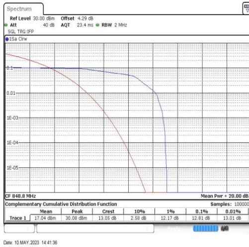
EGPRS850-251-8
