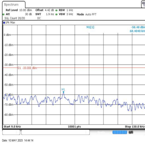
EGPRS850-190-8-0.009~0.15MHz-0.07
