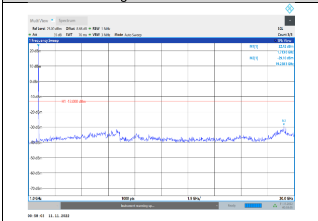
Band66-20MHz-QPSK-132072-1RB#0-Range2:1000~20000MHz
