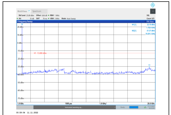
Band66-20MHz-QPSK-132322-1RB#0-Range2:1000~20000MHz
