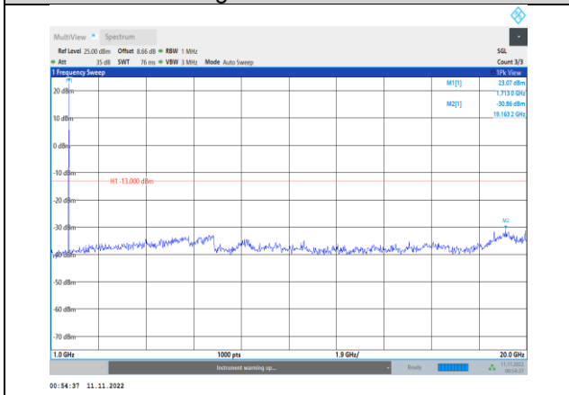
Band66-3MHz-QPSK-131987-1RB#0- Range2:1000~20000MHz
