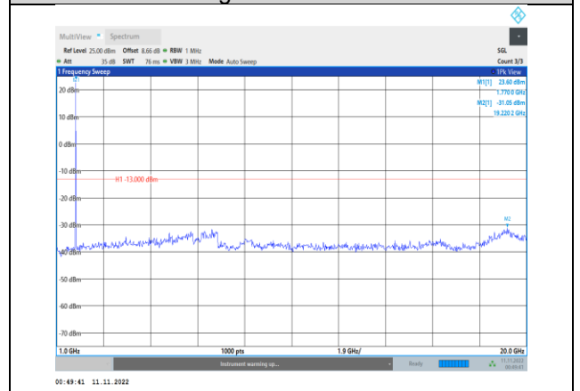
Band66-10MHz-QPSK-132622-1RB#0- Range2:1000~20000MHz
