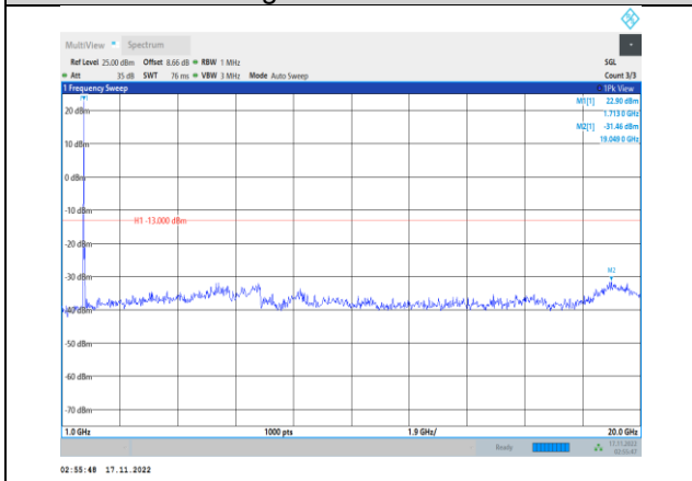
Band66-20MHz-64QAM-132072-1RB#0- Range2:1000~20000MHz
