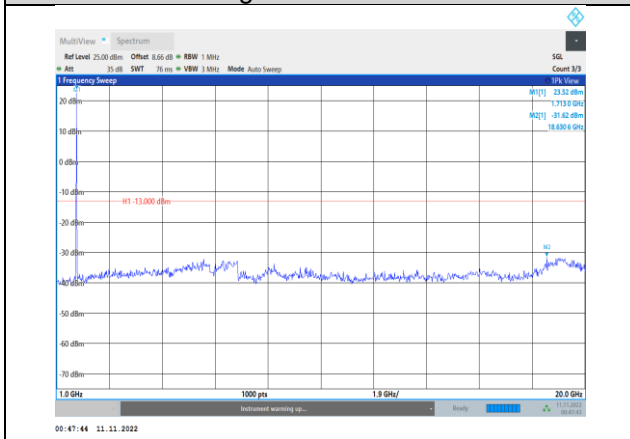
Band66-10MHz-QPSK-132022-1RB#0- Range2:1000~20000MHz
