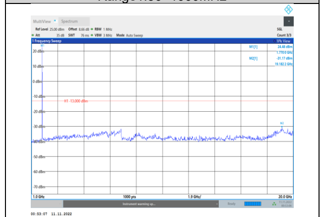
Band66-5MHz-QPSK-132647-1RB#0- Range2:1000~20000MHz
