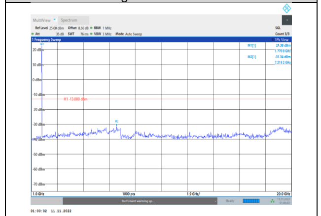
Band66-20MHz-QPSK-132572-1RB#0-Range2:1000~20000MHz
