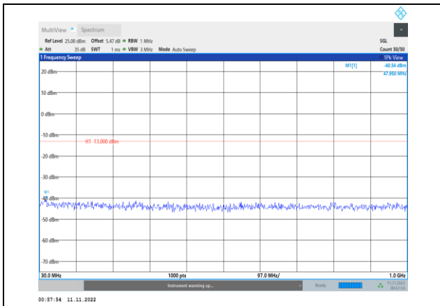
Band66-20MHz-QPSK-132072-1RB#0-Range1:30~1000MHz
