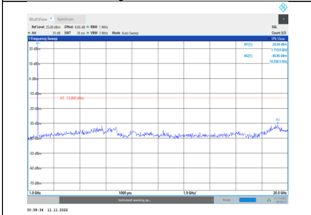
Band66-20MHz-16QAM-132072-1RB#0- Range2:1000~20000MHz
