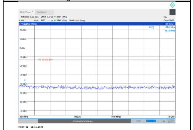
Band66-20MHz-QPSK-132572-1RB#0-Range1:30~1000MHz
