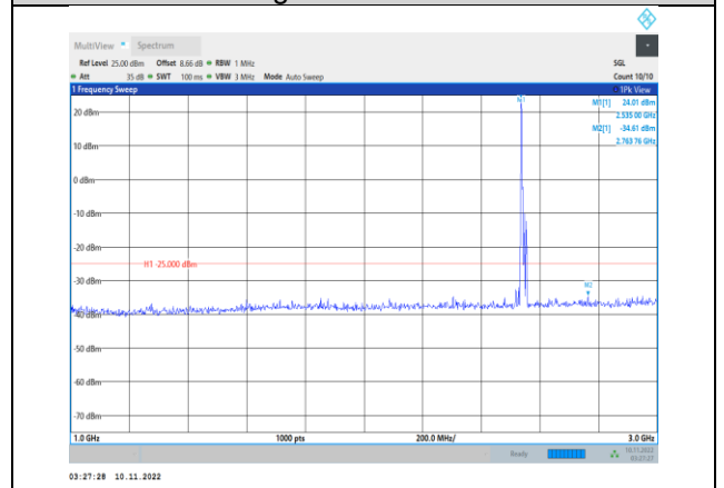
Band41-10MHz-QPSK-40090-1RB#0- Range2:1000~3000MHz
