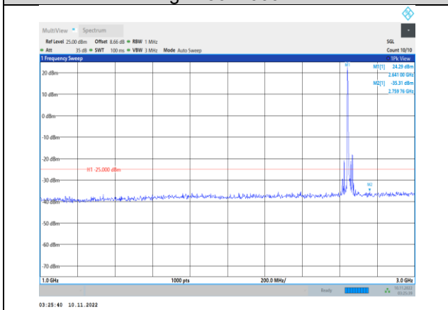
Band41-15MHz-QPSK-41165-1RB#0- Range2:1000~3000MHz
