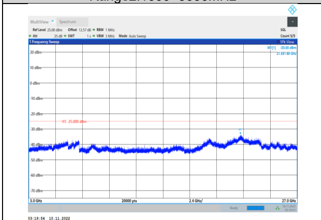
Band41-20MHz-QPSK-40640-1RB#0- Range3:3000~27000MHz
