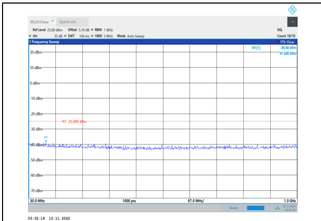
Band41-5MHz-QPSK-40065-1RB#0- Range1:30~1000MHz
