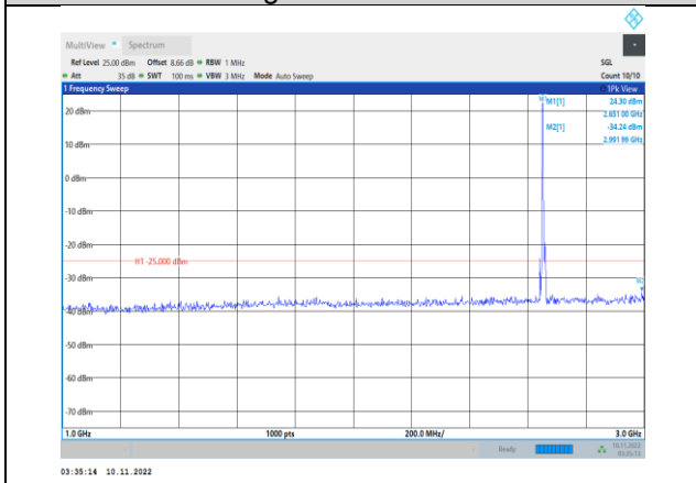
Band41-5MHz-QPSK-41215-1RB#0- Range2:1000~3000MHz
