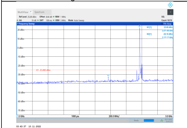
Band38-20MHz-16QAM-37850-1RB#0- Range2:1000~3000MHz
