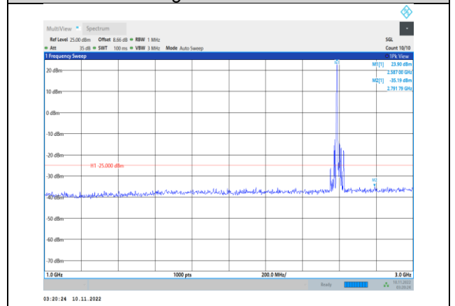
Band41-20MHz-16QAM-40640-1RB#0- Range2:1000~3000MHz
