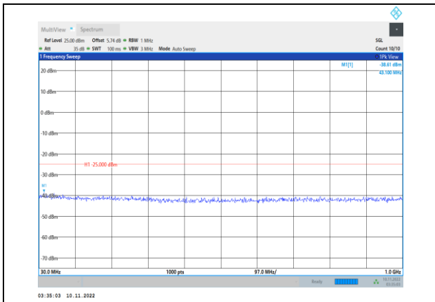
Band41-5MHz-QPSK-41215-1RB#0- Range1:30~1000MHz
