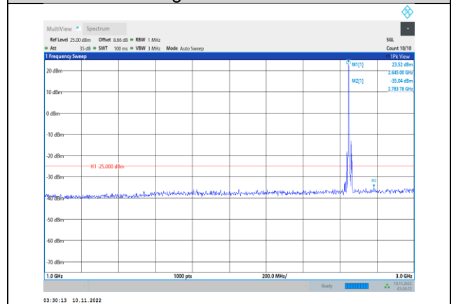
Band41-10MHz-QPSK-41190-1RB#0- Range2:1000~3000MHz
