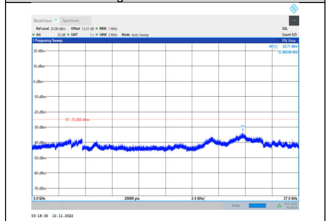
Band41-20MHz-QPSK-40140-1RB#0- Range3:3000~27000MHz
