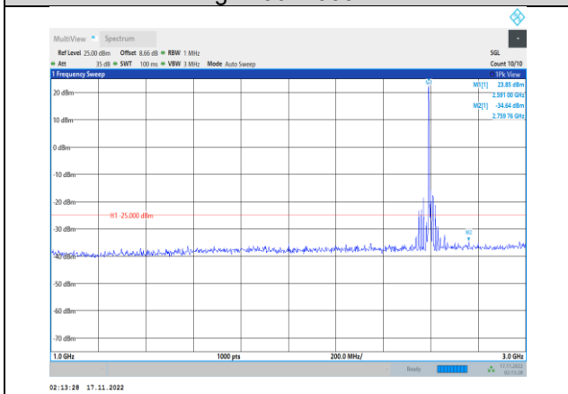
Band41-10MHz-64QAM-40640-1RB#0- Range2:1000~3000MHz
