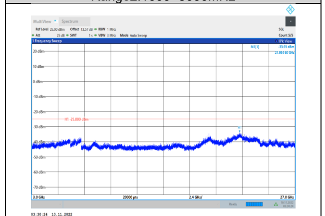
Band41-10MHz-QPSK-41190-1RB#0- Range3:3000~27000MHz
