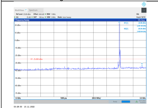
Band41-10MHz-QPSK-40640-1RB#0- Range2:1000~3000MHz
