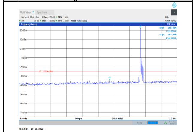
Band41-20MHz-QPSK-40140-1RB#0- Range2:1000~3000MHz
