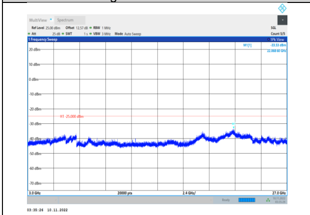
Band41-5MHz-QPSK-41215-1RB#0- Range3:3000~27000MHz
