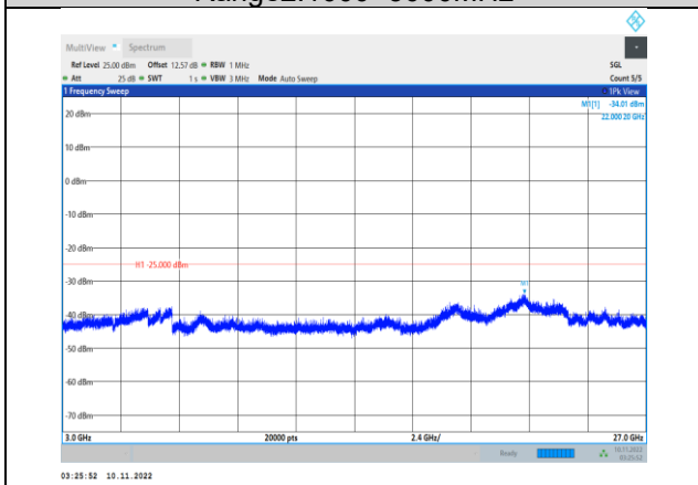
Band41-15MHz-QPSK-41165-1RB#0- Range3:3000~27000MHz
