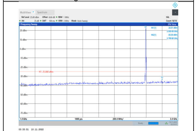
Band41-5MHz-QPSK-40640-1RB#0- Range2:1000~3000MHz
