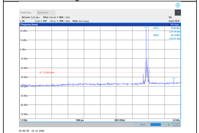
Band38-20MHz-QPSK-37850-1RB#0-Range2:1000~3000MHz
