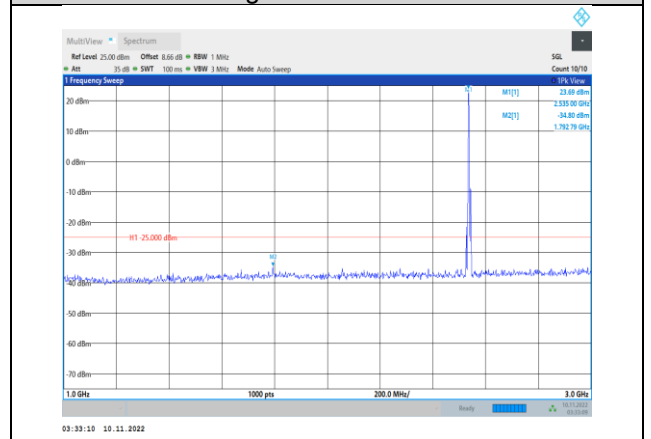
Band41-5MHz-16QAM-40065-1RB#0- Range2:1000~3000MHz
