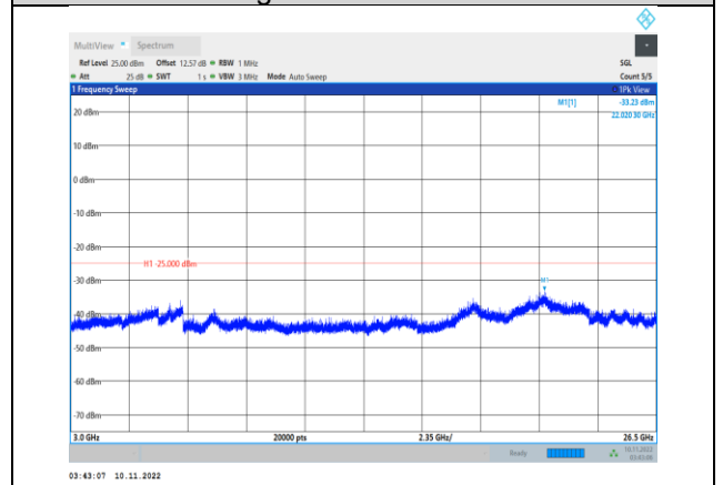
Band38-20MHz-QPSK-37850-1RB#0-Range3:3000~26500MHz
