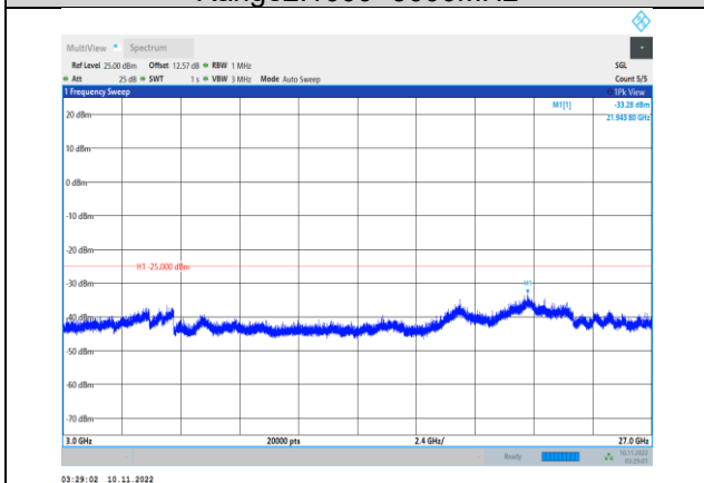
Band41-10MHz-QPSK-40640-1RB#0- Range3:3000~27000MHz
