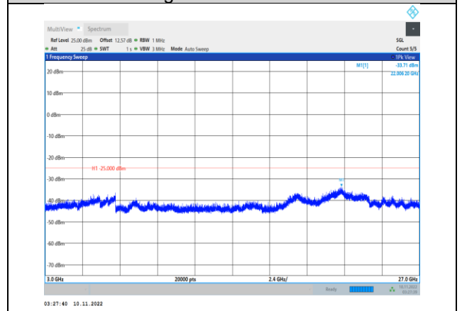
Band41-10MHz-QPSK-40090-1RB#0- Range3:3000~27000MHz
