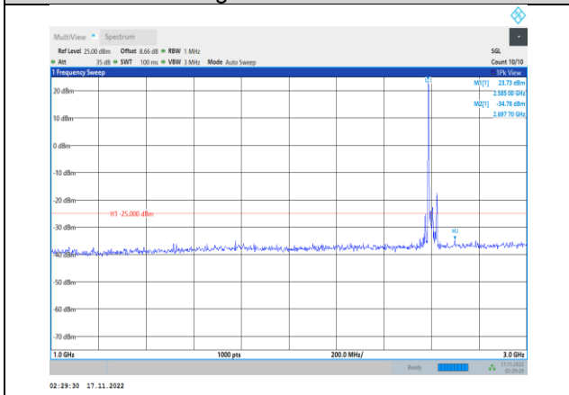
Band41-20MHz-64QAM-40640-1RB#0- Range2:1000~3000MHz
