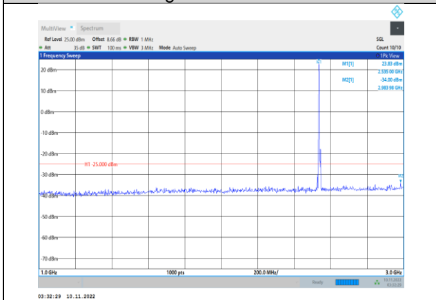
Band41-5MHz-QPSK-40065-1RB#0- Range2:1000~3000MHz
