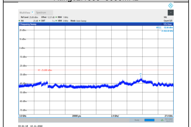
Band41-20MHz-QPSK-41140-1RB#0- Range3:3000~27000MHz
