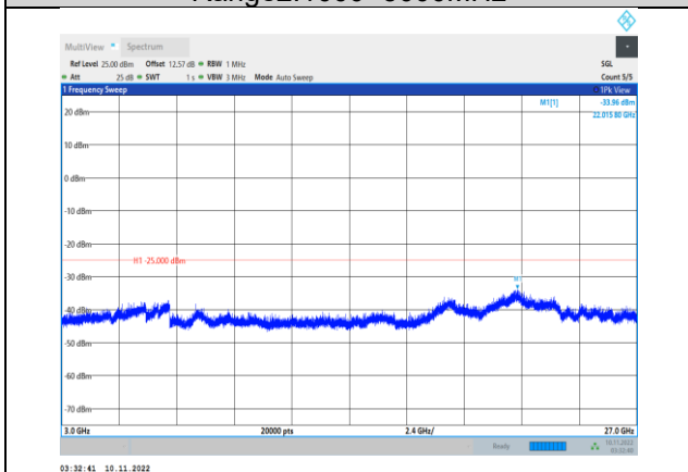
Band41-5MHz-QPSK-40065-1RB#0- Range3:3000~27000MHz
