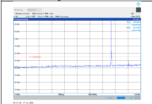
Band41-5MHz-64QAM-40065-1RB#0- Range2:1000~3000MHz
