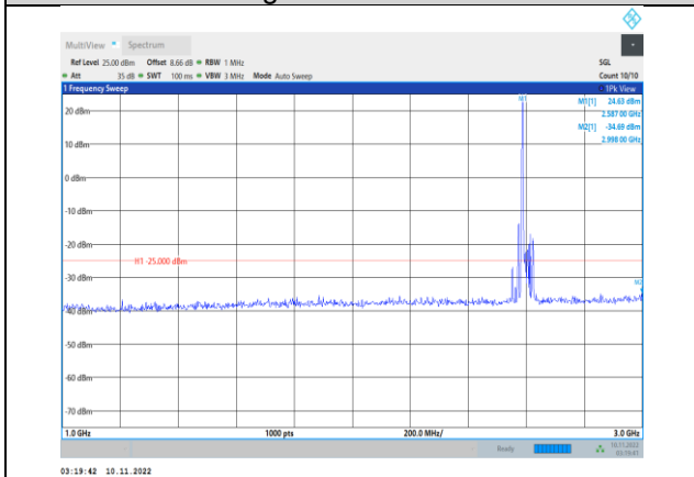
Band41-20MHz-QPSK-40640-1RB#0- Range2:1000~3000MHz
