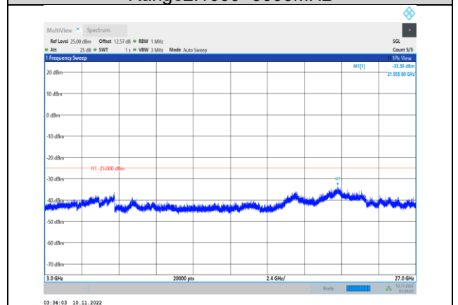
Band41-5MHz-QPSK-40640-1RB#0- Range3:3000~27000MHz
