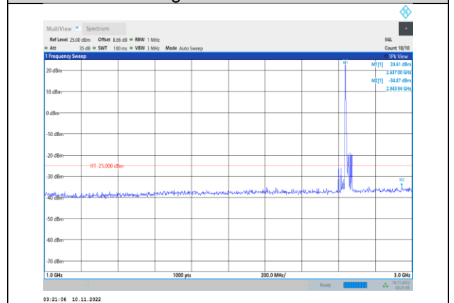
Band41-20MHz-QPSK-41140-1RB#0- Range2:1000~3000MHz
