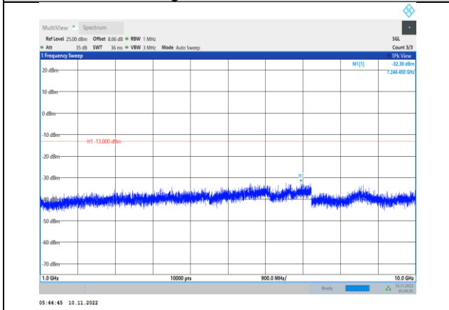
Band26-5MHz-QPSK-26715-1RB#0- Range2:1000~10000MHz
