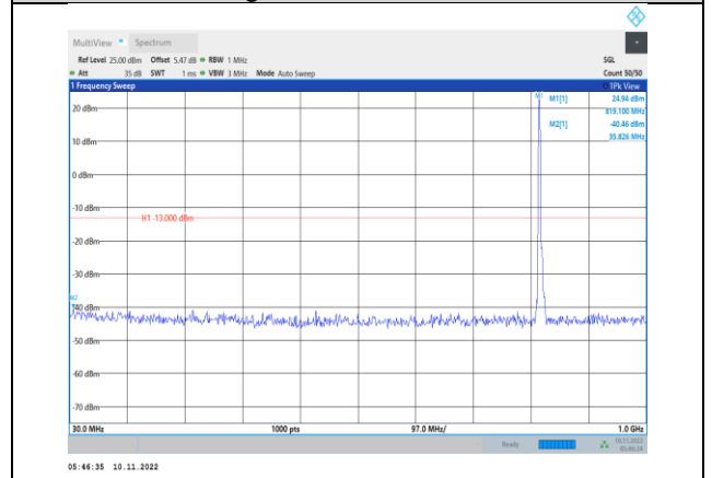
Band26-5MHz-QPSK-26765-1RB#0- Range1:30~1000MHz
