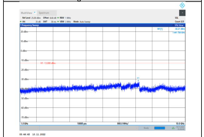
Band26-5MHz-QPSK-26765-1RB#0- Range2:1000~10000MHz
