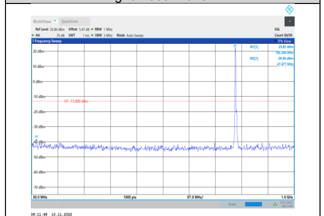
Band13-5MHz-QPSK-23255-1RB#0- Range1:30~1000MHz
