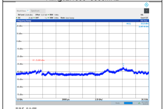
Band7-5MHz-QPSK-21100-1RB#0- Range3:3000~26500MHz
