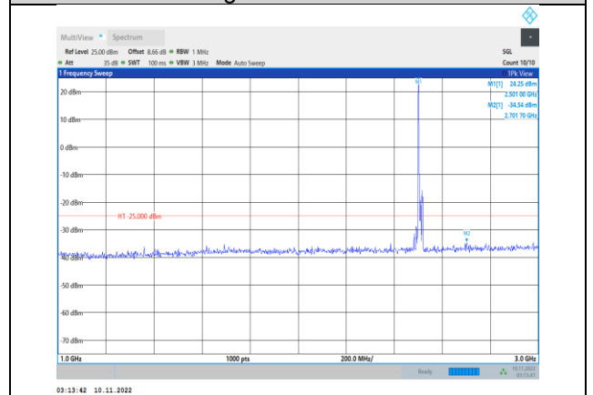
Band7-10MHz-QPSK-20800-1RB#0- Range2:1000~3000MHz
