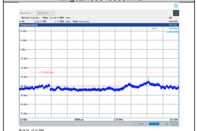
Band7-15MHz-QPSK-20825-1RB#0- Range3:3000~26500MHz
