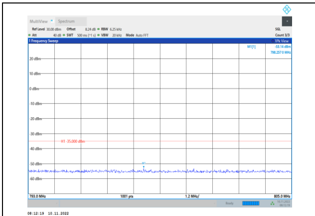
Band13-5MHz-QPSK-23255-1RB#0-Range4:793~805MHz
