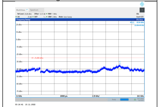
Band7-10MHz-QPSK-21400-1RB#0- Range3:3000~26500MHz
