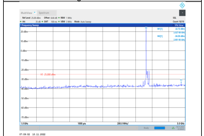
Band7-20MHz-QPSK-21100-1RB#0- Range2:1000~3000MHz
