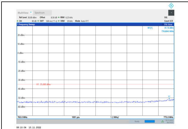
Band13-5MHz-QPSK-23230-1RB#0- Range3:763~775MHz
