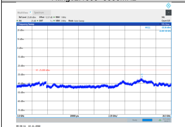
Band7-5MHz-QPSK-21425-1RB#0- Range3:3000~26500MHz
