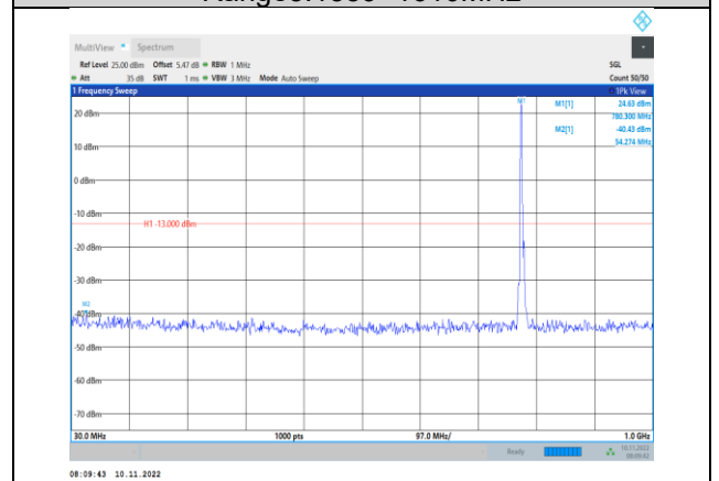
Band13-5MHz-QPSK-23230-1RB#0- Range1:30~1000MHz
