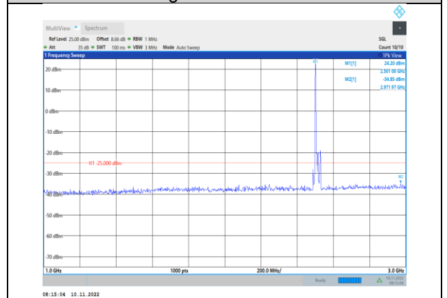
Band7-15MHz-QPSK-20825-1RB#0- Range2:1000~3000MHz
