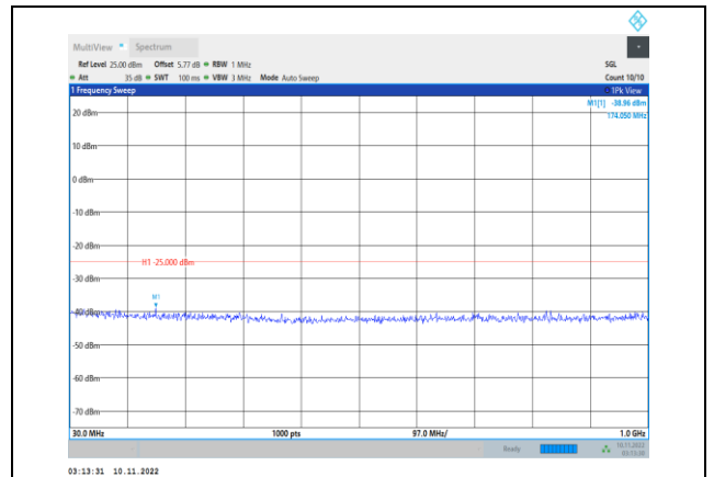
Band7-10MHz-QPSK-20800-1RB#0- Range1:30~1000MHz
