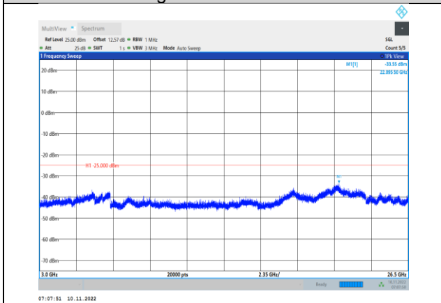
Band7-20MHz-QPSK-20850-1RB#0- Range3:3000~26500MHz
