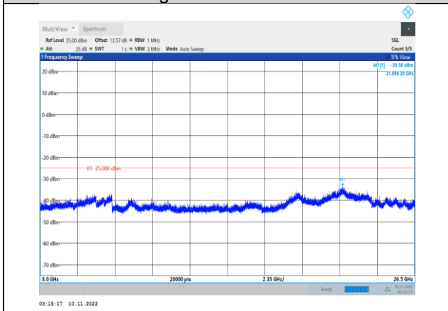
Band7-10MHz-QPSK-21100-1RB#0- Range3:3000~26500MHz
