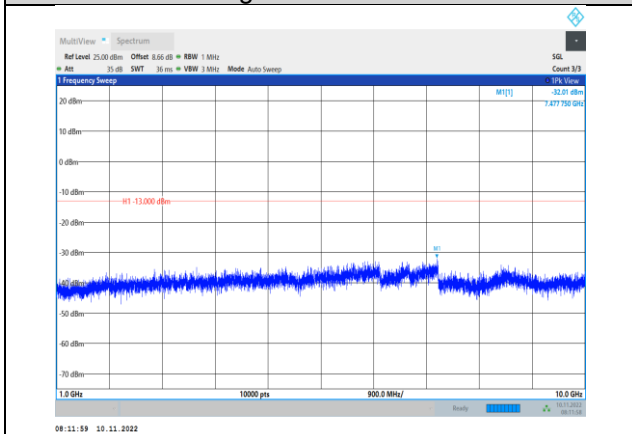
Band13-5MHz-QPSK-23255-1RB#0-Range2:1000~10000MHz
