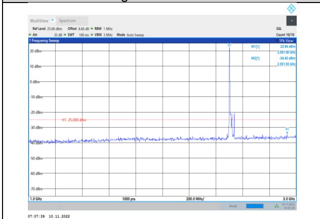
Band7-20MHz-QPSK-20850-1RB#0- Range2:1000~3000MHz
