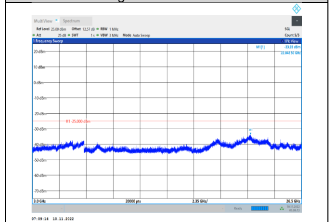
Band7-20MHz-QPSK-21100-1RB#0- Range3:3000~26500MHz
