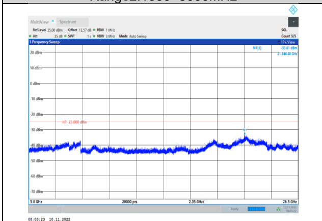
Band7-5MHz-QPSK-20775-1RB#0- Range3:3000~26500MHz
