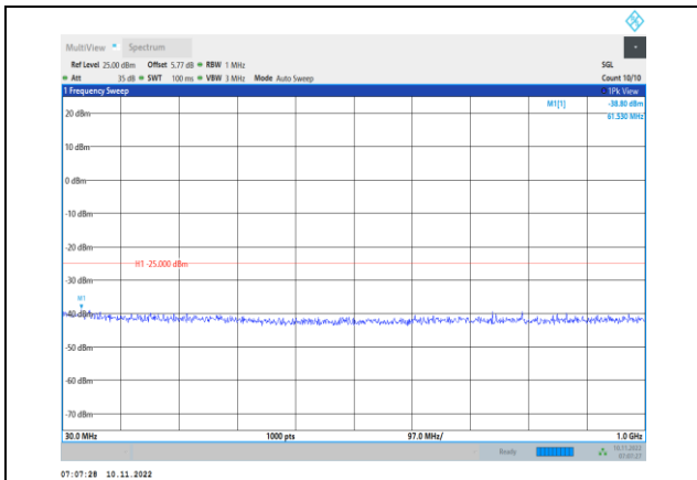
Band7-20MHz-QPSK-20850-1RB#0- Range1:30~1000MHz
