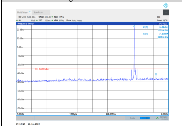
Band7-20MHz-QPSK-21350-1RB#0-Range2:1000~3000MHz
