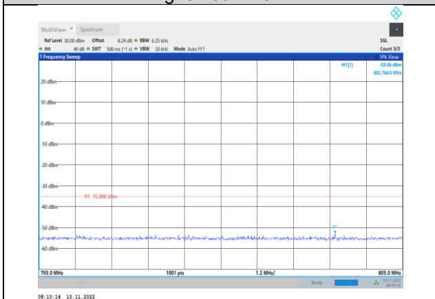
Band13-5MHz-QPSK-23230-1RB#0- Range4:793~805MHz
