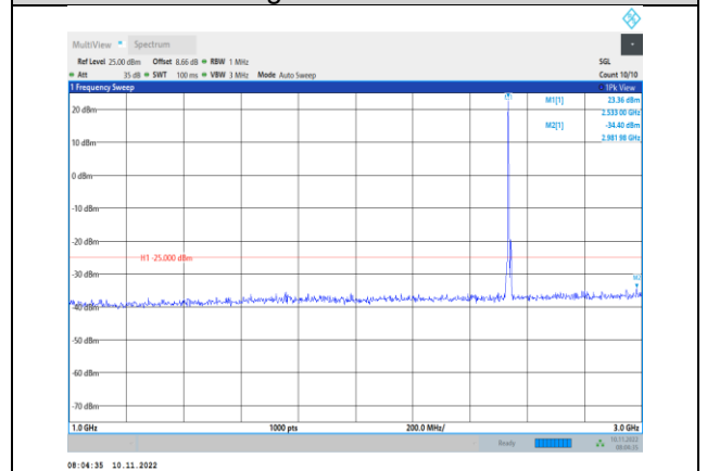
Band7-5MHz-QPSK-21100-1RB#0- Range2:1000~3000MHz
