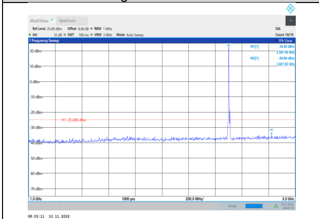
Band7-5MHz-QPSK-20775-1RB#0- Range2:1000~3000MHz
