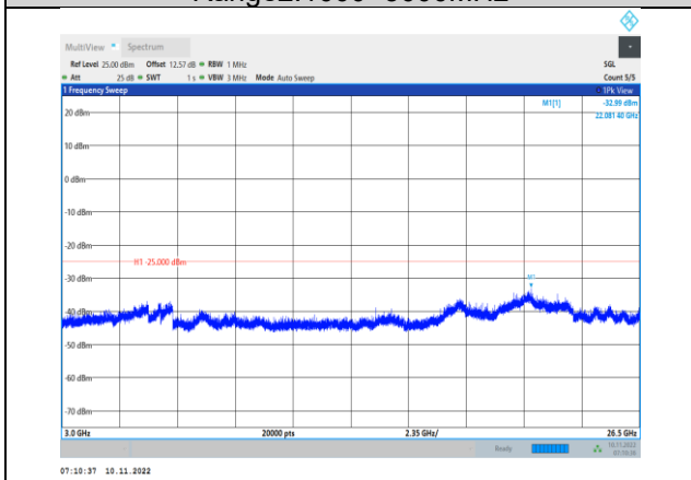
Band7-20MHz-QPSK-21350-1RB#0-Range3:3000~26500MHz
