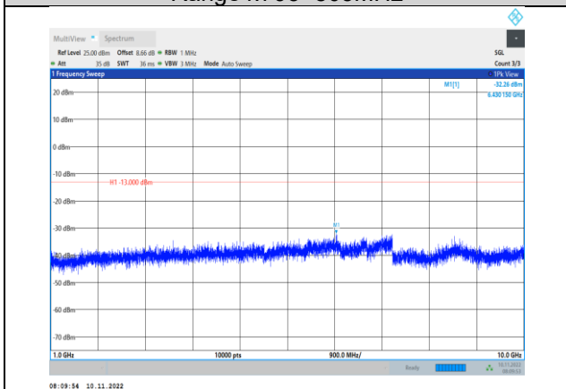
Band13-5MHz-QPSK-23230-1RB#0- Range2:1000~10000MHz
