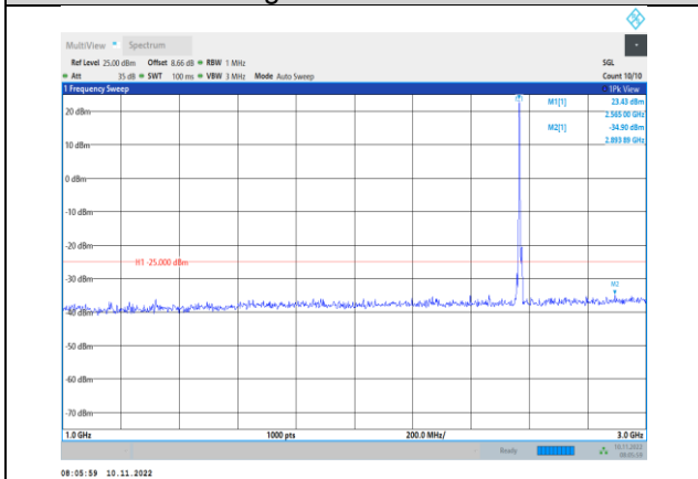
Band7-5MHz-QPSK-21425-1RB#0- Range2:1000~3000MHz
