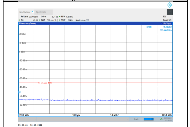
Band13-10MHz-QPSK-23230-1RB#0- Range4:793~805MHz
