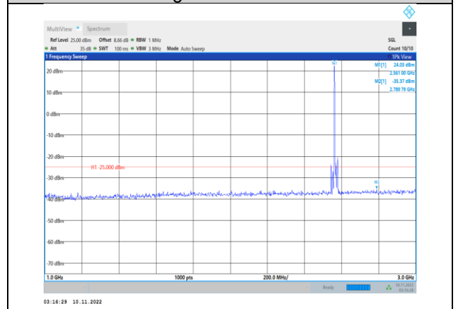
Band7-10MHz-QPSK-21400-1RB#0- Range2:1000~3000MHz
