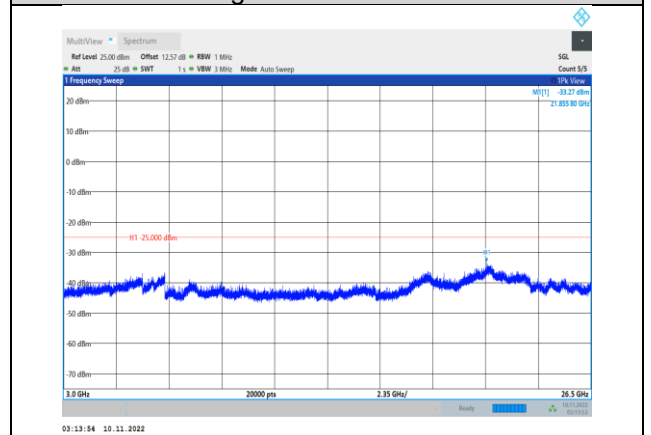
Band7-10MHz-QPSK-20800-1RB#0- Range3:3000~26500MHz
