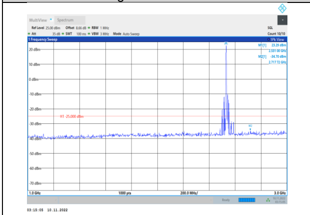
Band7-10MHz-QPSK-21100-1RB#0- Range2:1000~3000MHz
