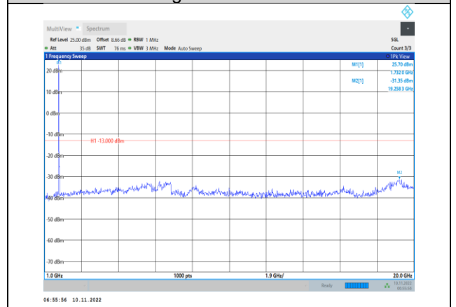
Band4-20MHz-QPSK-20300-1RB#0- Range2:1000~20000MHz
