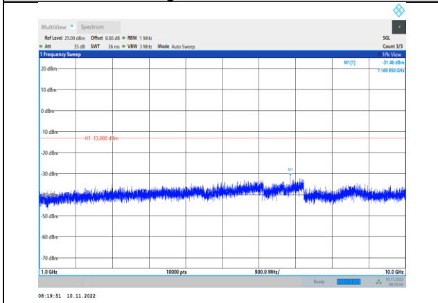
Band5-5MHz-QPSK-20425-1RB#0- Range2:1000~10000MHz
