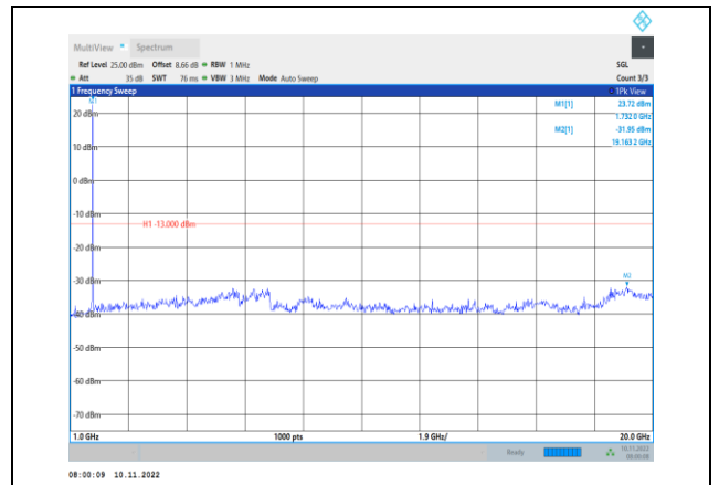
Band4-5MHz-QPSK-20175-1RB#0- Range2:1000~20000MHz
