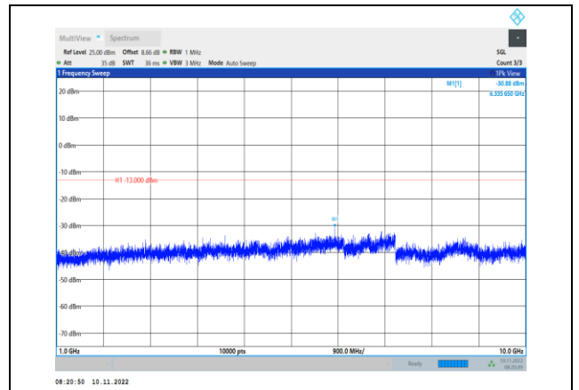
Band5-5MHz-QPSK-20525-1RB#0- Range2:1000~10000MHz
