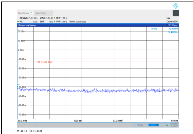
Band4-10MHz-QPSK-20000-1RB#0-Range1:30~1000MHz
