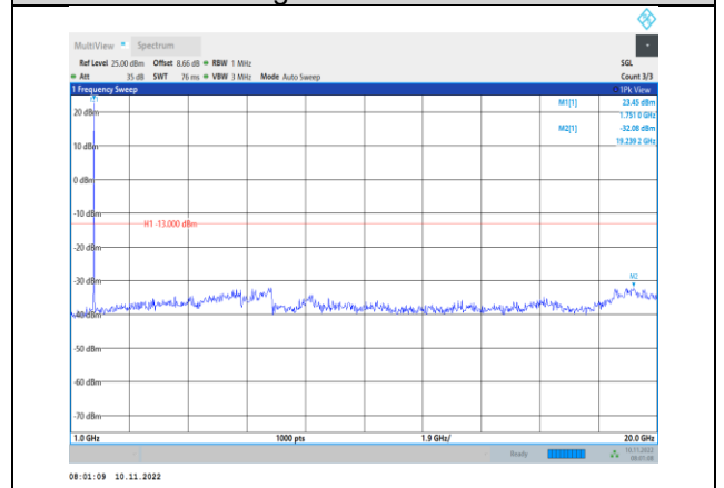
Band4-5MHz-QPSK-20375-1RB#0- Range2:1000~20000MHz
