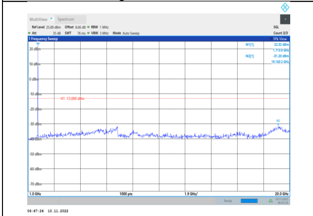
Band4-15MHz-QPSK-20025-1RB#0-Range2:1000~20000MHz
