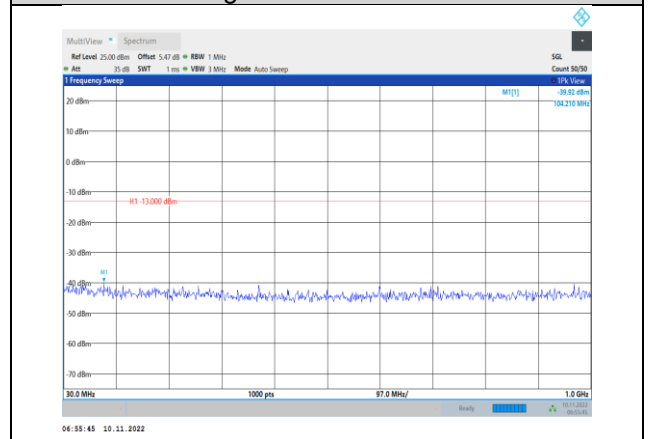
Band4-20MHz-QPSK-20300-1RB#0- Range1:30~1000MHz
