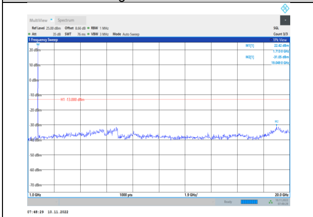
Band4-10MHz-QPSK-20000-1RB#0-Range2:1000~20000MHz
