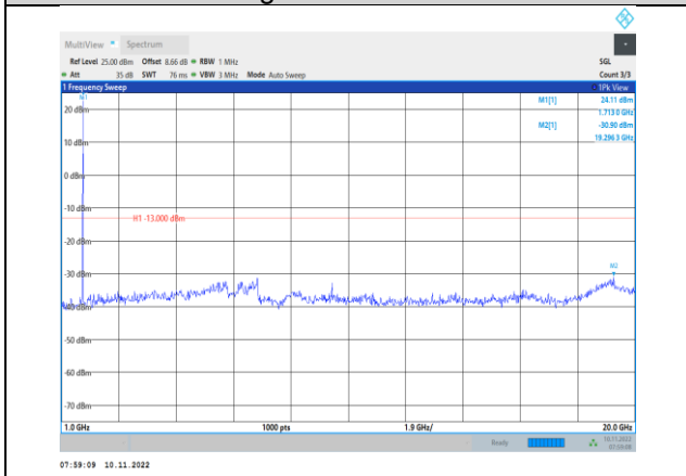
Band4-5MHz-QPSK-19975-1RB#0- Range2:1000~20000MHz
