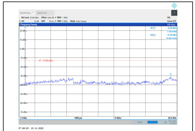
Band4-10MHz-QPSK-20175-1RB#0-Range2:1000~20000MHz
