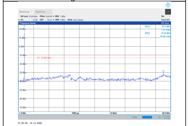
Band4-10MHz-QPSK-20350-1RB#0-Range2:1000~20000MHz
