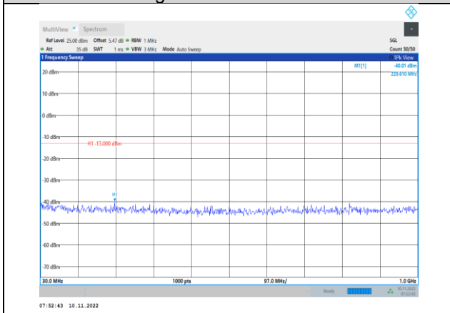
Band2-20MHz-QPSK-18900-1RB#0-Range1:30~1000MHz
