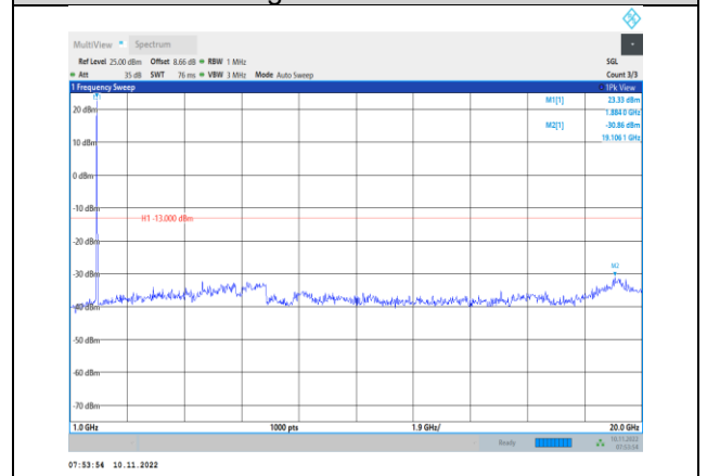
Band2-20MHz-QPSK-19100-1RB#0-Range2:1000~20000MHz
