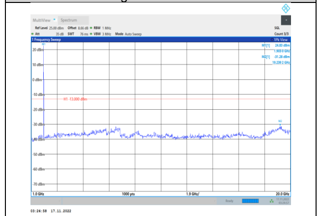
Band2-5MHz-64QAM-19175-1RB#0- Range2:1000~20000MHz
