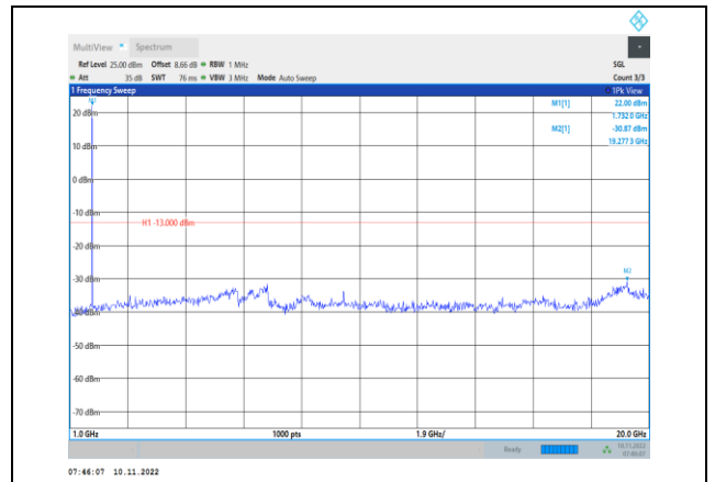
Band4-3MHz-QPSK-20175-1RB#0- Range2:1000~20000MHz
