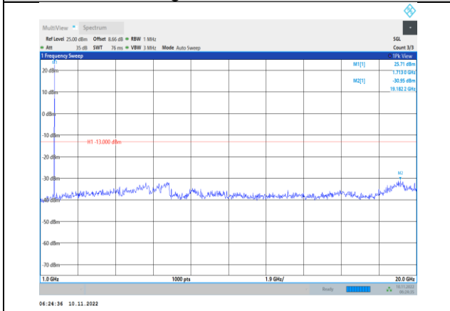
Band4-1.4MHz-QPSK-19957-1RB#0-Range2:1000~20000MHz
