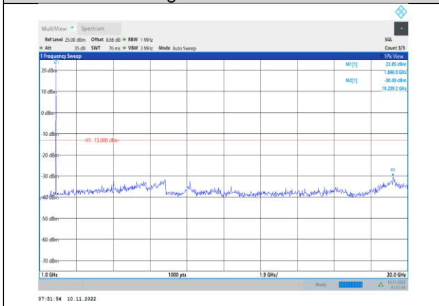
Band2-20MHz-QPSK-18700-1RB#0-Range2:1000~20000MHz
