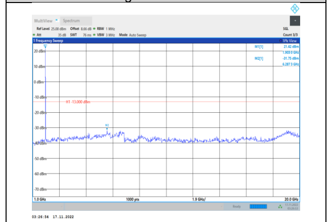
Band2-3MHz-64QAM-19185-1RB#0-Range2:1000~20000MHz
