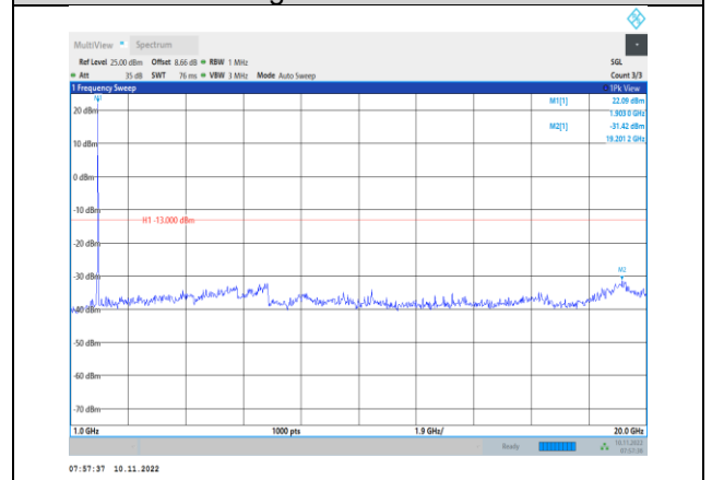
Band2-15MHz-QPSK-19125-1RB#0-Range2:1000~20000MHz
