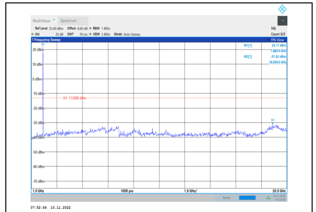
Band2-20MHz-QPSK-18900-1RB#0-Range2:1000~20000MHz
