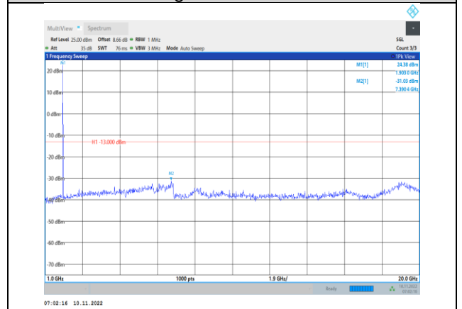
Band2-1.4MHz-QPSK-19193-1RB#0- Range2:1000~20000MHz
