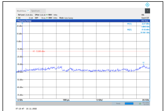
Band2-3MHz-QPSK-18900-1RB#0- Range2:1000~20000MHz
