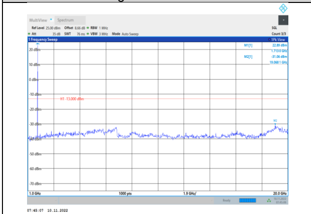
Band4-3MHz-QPSK-19965-1RB#0- Range2:1000~20000MHz
