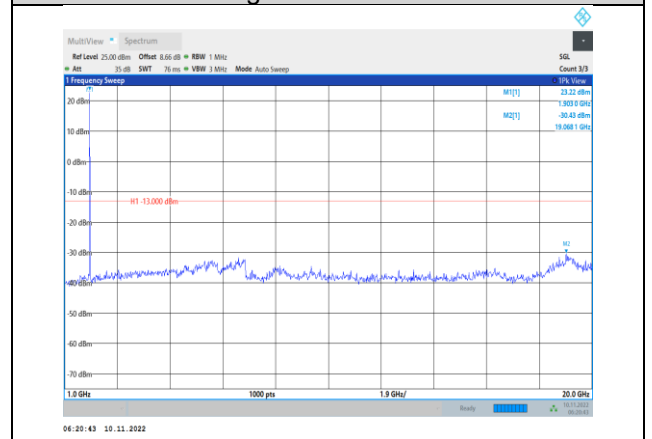
Band2-5MHz-QPSK-19175-1RB#0- Range2:1000~20000MHz
