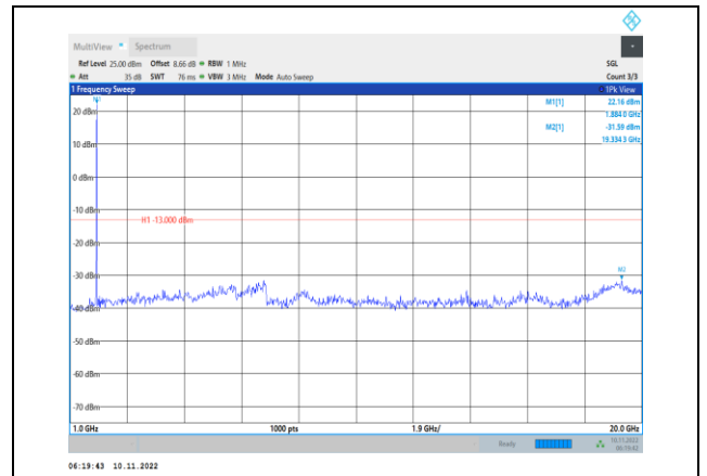
Band2-5MHz-QPSK-18900-1RB#0- Range2:1000~20000MHz
