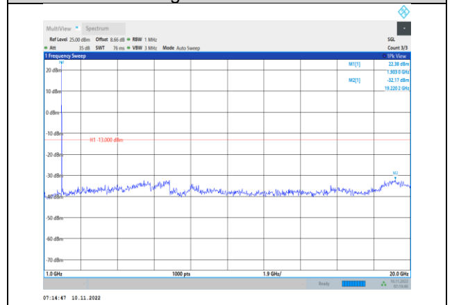
Band2-3MHz-QPSK-19185-1RB#0- Range2:1000~20000MHz
