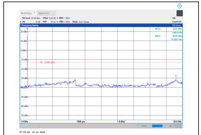
Band2-20MHz-16QAM-18900-1RB#0- Range2:1000~20000MHz
