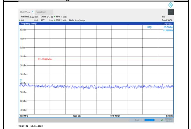
Band2-5MHz-QPSK-19175-1RB#0- Range1:30~1000MHz
