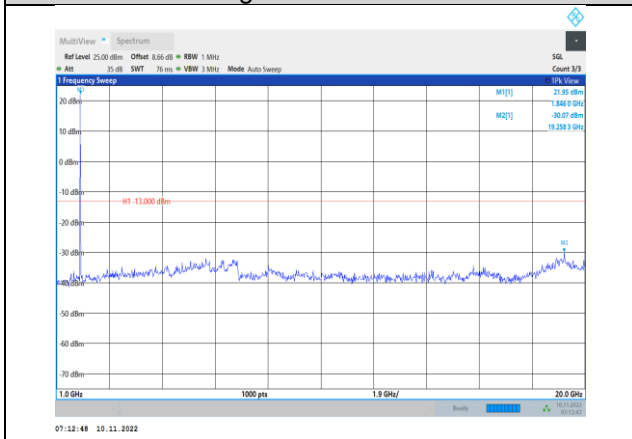
Band2-3MHz-QPSK-18615-1RB#0- Range2:1000~20000MHz
