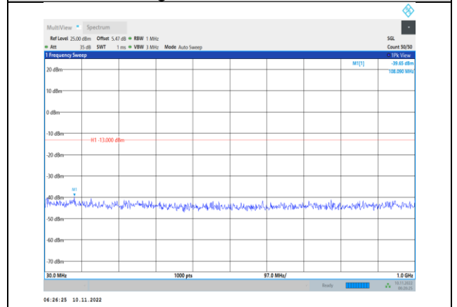
Band4-1.4MHz-QPSK-20393-1RB#0-Range1:30~1000MHz
