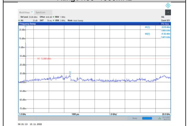
Band2-5MHz-16QAM-19175-1RB#0- Range2:1000~20000MHz
