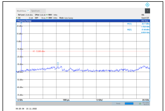
Band4-1.4MHz-QPSK-20175-1RB#0-Range2:1000~20000MHz
