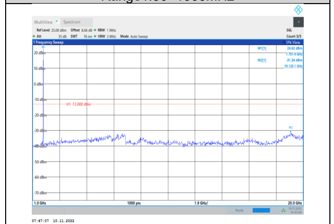
Band4-3MHz-QPSK-20385-1RB#0- Range2:1000~20000MHz
