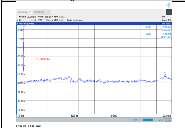
Band2-20MHz-16QAM-18700-1RB#0- Range2:1000~20000MHz
