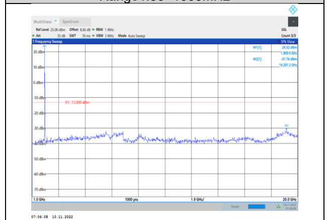
Band2-10MHz-QPSK-19150-1RB#0- Range2:1000~20000MHz
