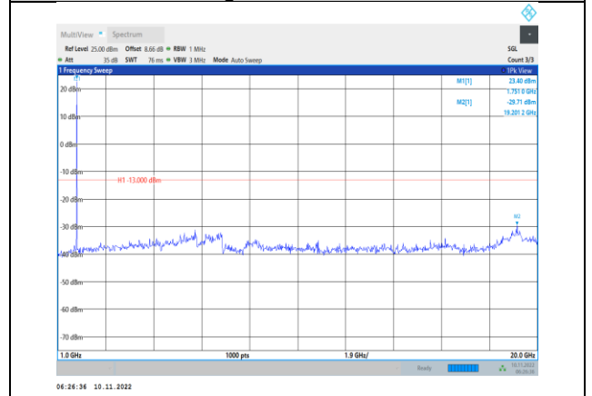
Band4-1.4MHz-QPSK-20393-1RB#0-Range2:1000~20000MHz
