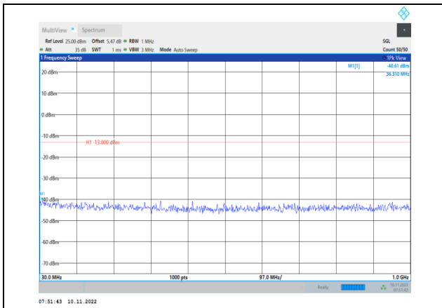
Band2-20MHz-QPSK-18700-1RB#0-Range1:30~1000MHz
