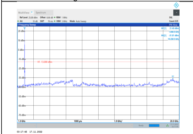
Band2-20MHz-64QAM-18700-1RB#0- Range2:1000~20000MHz
