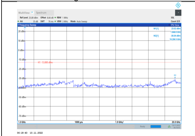
Band2-5MHz-QPSK-18625-1RB#0- Range2:1000~20000MHz
