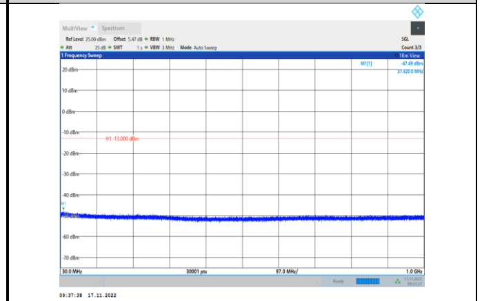
GPRS1900-810-0-30~1000MHz
