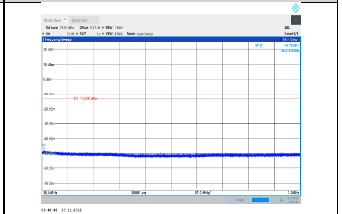
EGPRS1900-810-2-30~1000MHz
