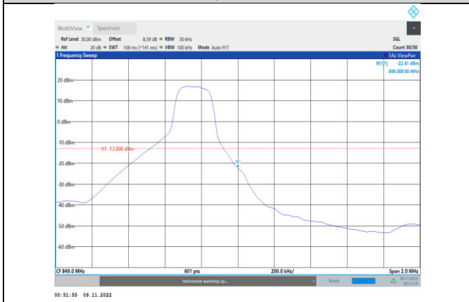
Band5-3MHz-QPSK-20635-1RB#14
