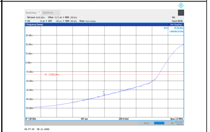
Band2-20MHz-16QAM-18700-1RB#0
