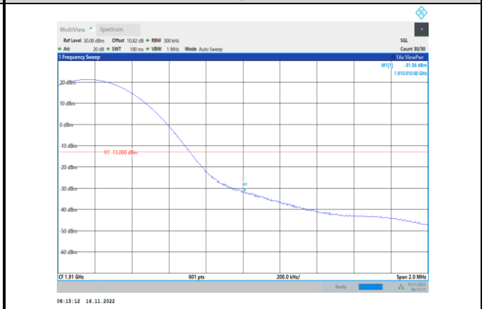
Band2-15MHz-64QAM-19125-1RB#74
