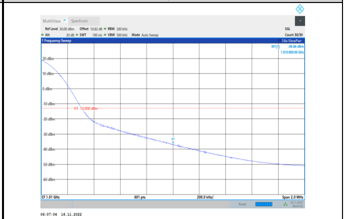
Band2-20MHz-64QAM-19100-1RB#99
