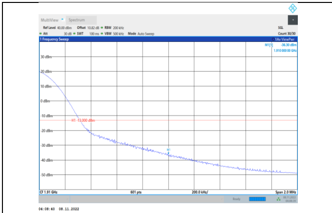
Band2-20MHz-16QAM-19100-1RB#99
