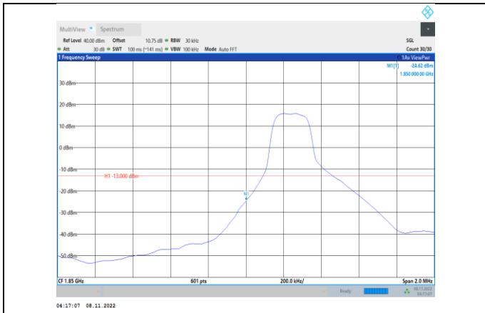
Band2-3MHz-QPSK-18615-1RB#0
