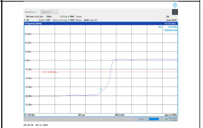
Band2-3MHz-16QAM-18615-15RB#0
