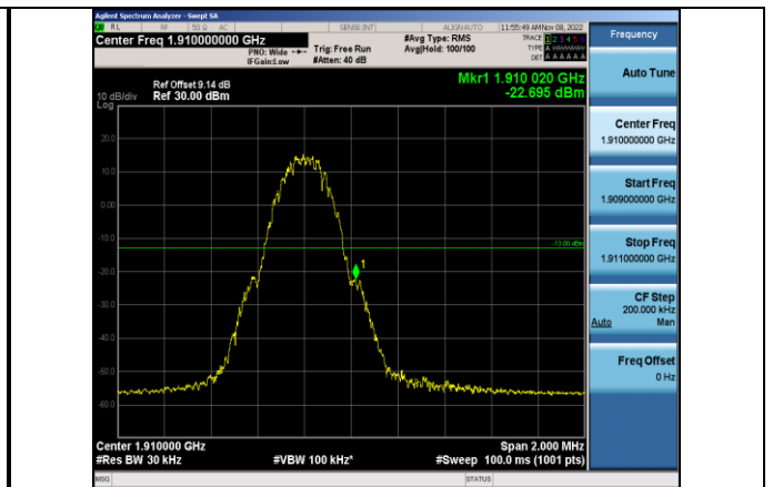
GPRS1900-810-0
