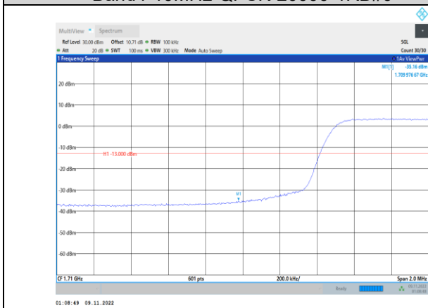
Band4-10MHz-QPSK-20000-50RB#0
