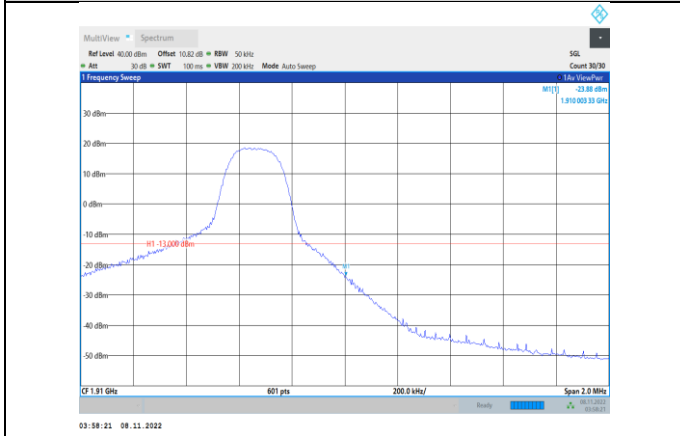
Band2-5MHz-QPSK-19175-1RB#24
