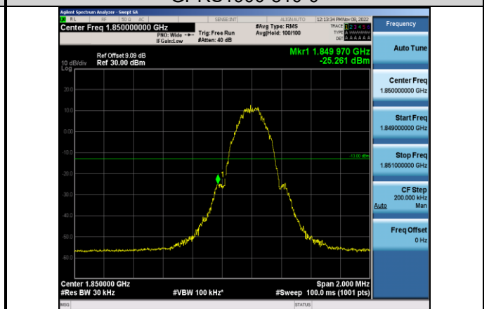
EGPRS1900-512-2
