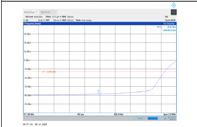
Band2-20MHz-QPSK-18700-100RB#0
