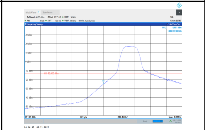
Band2-5MHz-16QAM-18625-1RB#0
