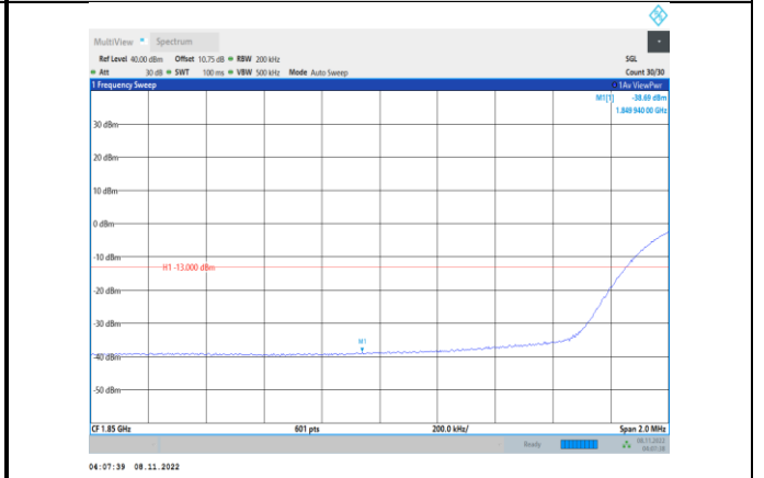
Band2-20MHz-16QAM-18700-100RB#0
