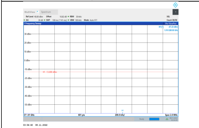
Band2-3MHz-QPSK-19185-1RB#14
