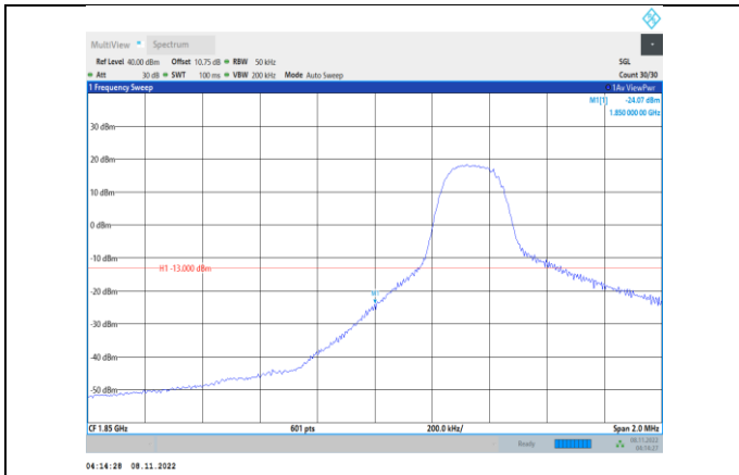
Band2-5MHz-QPSK-18625-1RB#0
