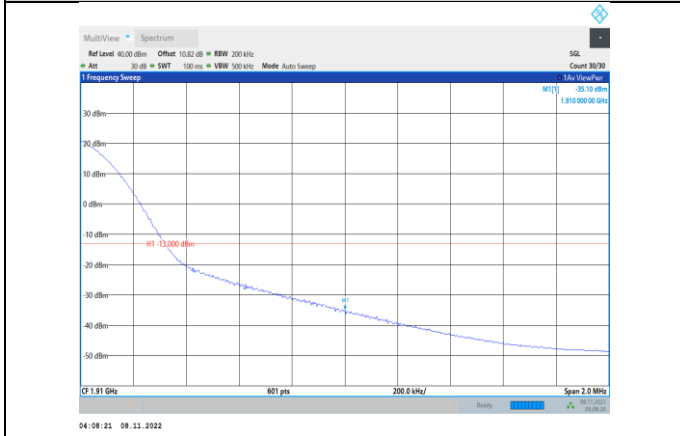
Band2-20MHz-QPSK-19100-1RB#99
