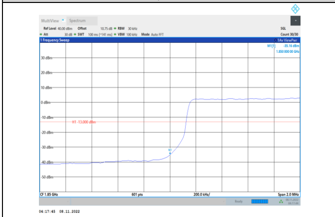
Band2-3MHz-QPSK-18615-15RB#0
