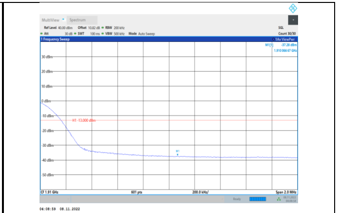
Band2-20MHz-QPSK-19100-100RB#0
