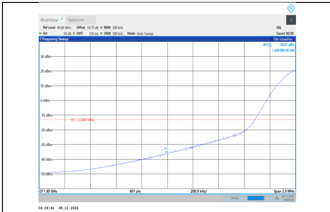
Band2-20MHz-QPSK-18700-1RB#0
