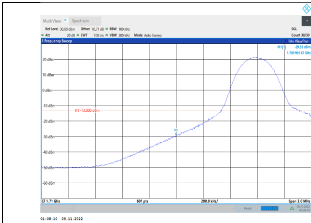
Band4-10MHz-QPSK-20000-1RB#0
