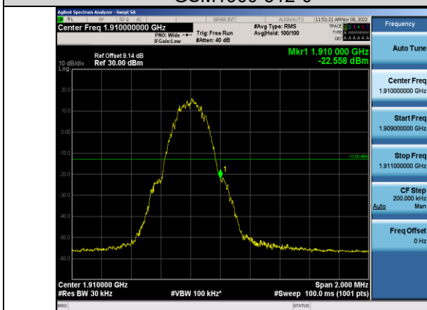
GSM1900-810-0
