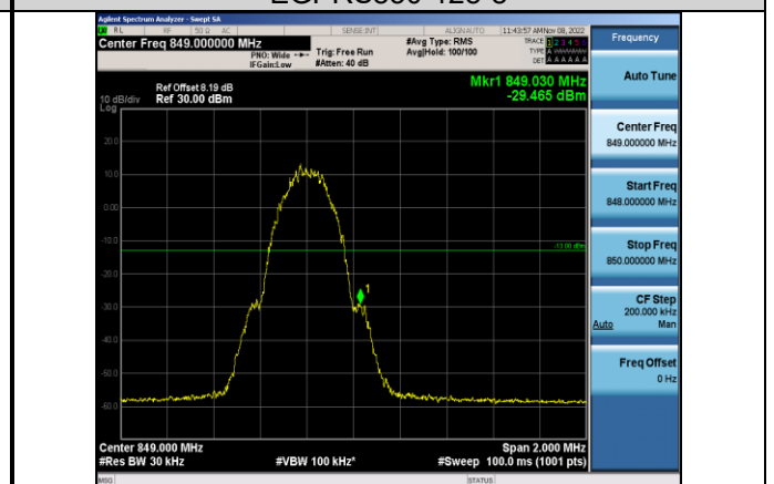
EGPRS850-251-8
