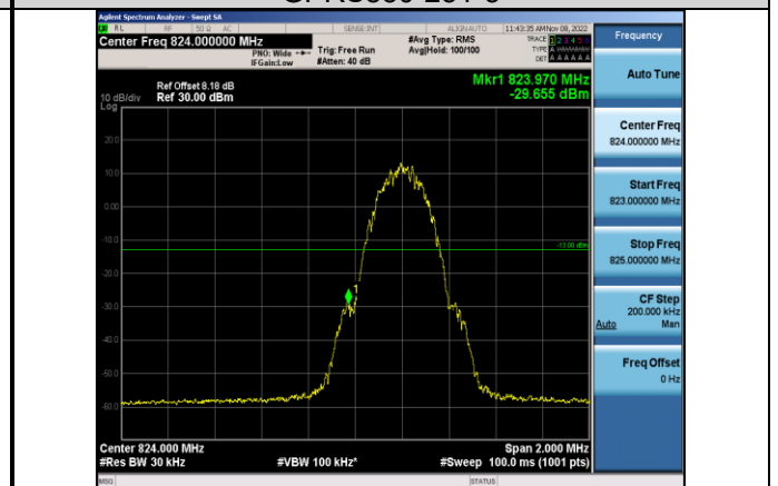
EGPRS850-128-8
