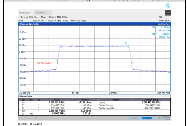
Band41-10MHz-QPSK-40640-50RB#0
