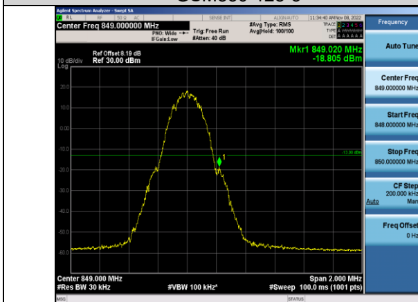
GSM850-251-3
