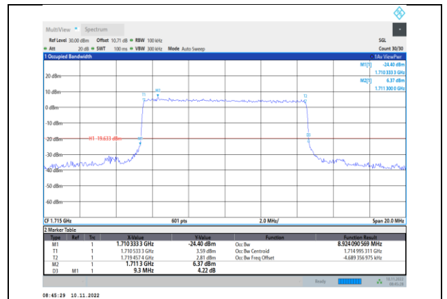
Band66-10MHz-QPSK-132022-50RB#0
