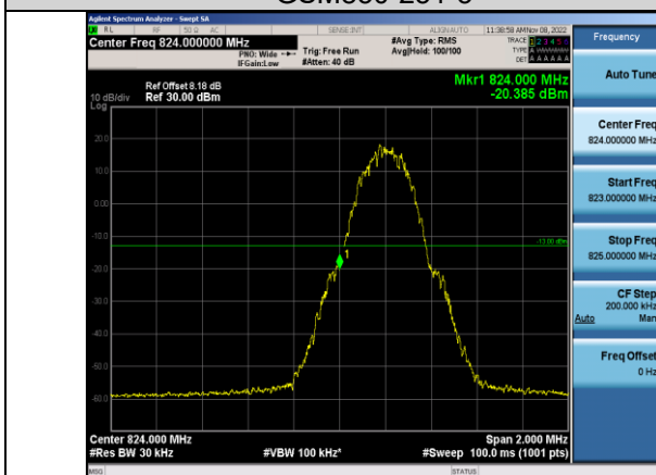
GPRS850-128-3
