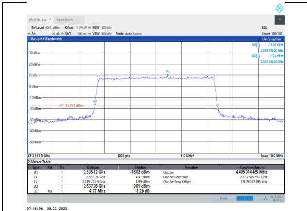
Band41-5MHz-QPSK-40065-25RB#0
