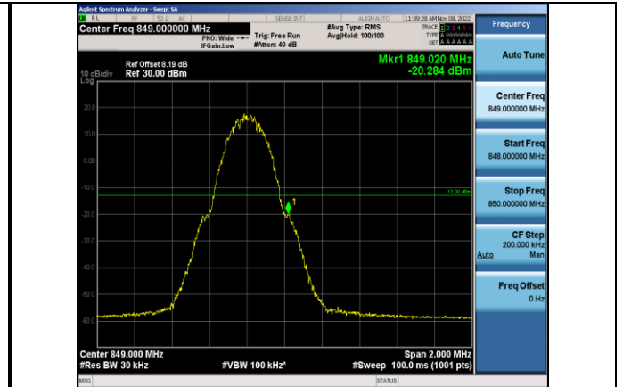
GPRS850-251-3
