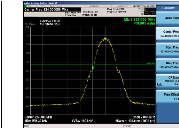
GSM850-128-3
