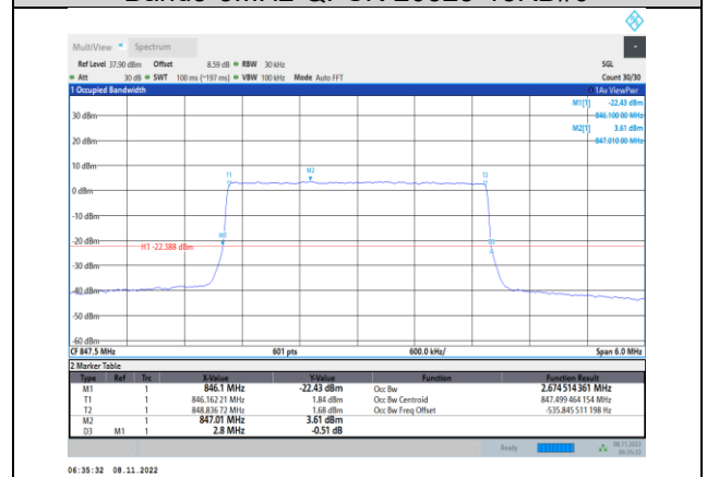
Band5-3MHz-QPSK-20635-15RB#0
