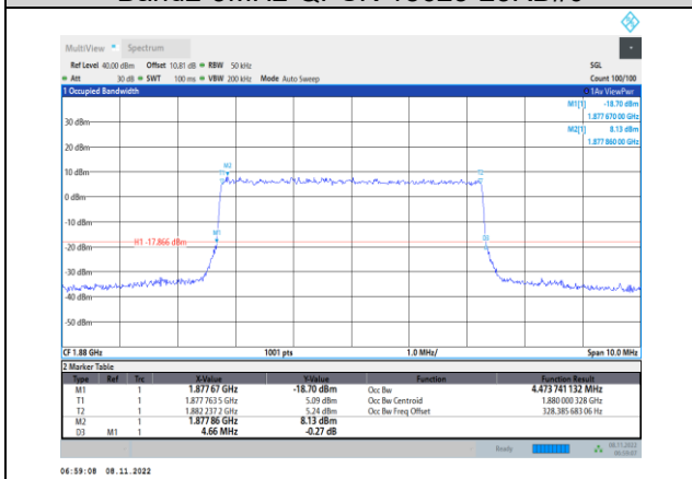
Band2-5MHz-QPSK-18900-25RB#0
