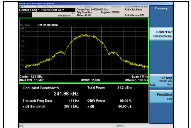
EGPRS1900-512-2-0.2979
