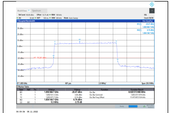
Band2-10MHz-QPSK-18650-50RB#0
