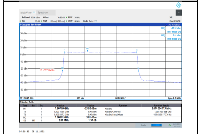
Band2-3MHz-QPSK-19185-15RB#0
