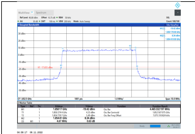
Band2-5MHz-QPSK-18625-25RB#0
