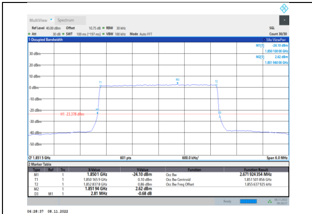
Band2-3MHz-16QAM-18615-15RB#0
