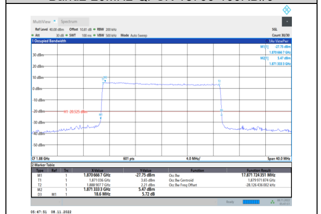
Band2-20MHz-QPSK-18900-100RB#0
