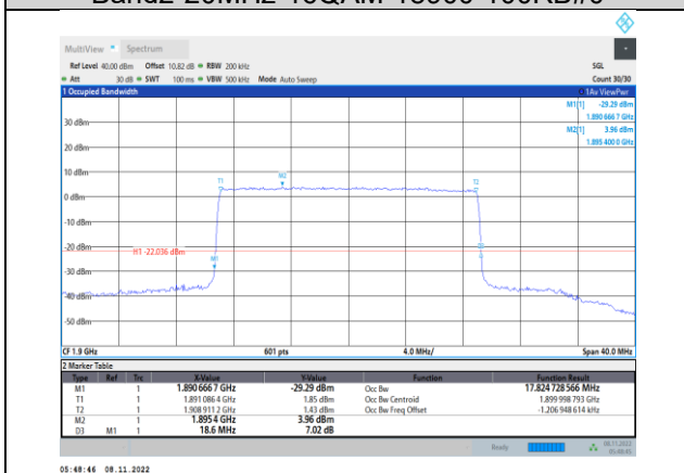
Band2-20MHz-16QAM-19100-100RB#0
