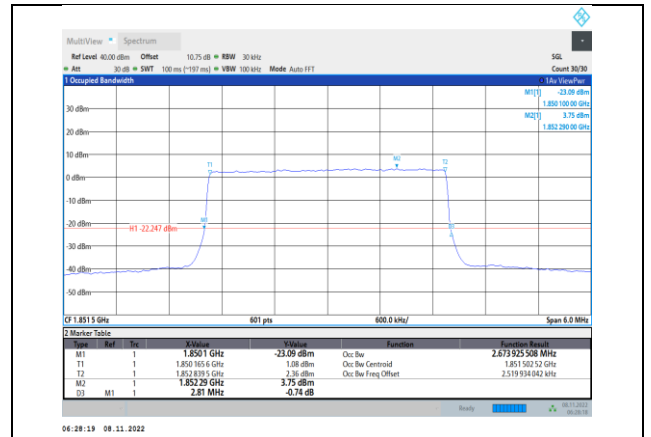
Band2-3MHz-QPSK-18615-15RB#0
