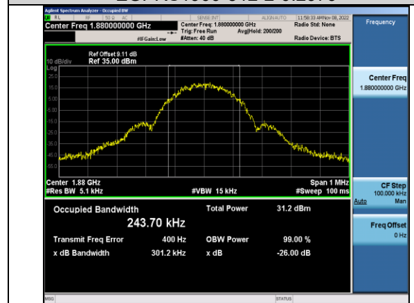
EGPRS1900-661-2-0.3012
