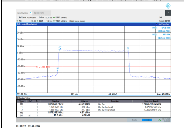
Band2-20MHz-16QAM-18900-100RB#0
