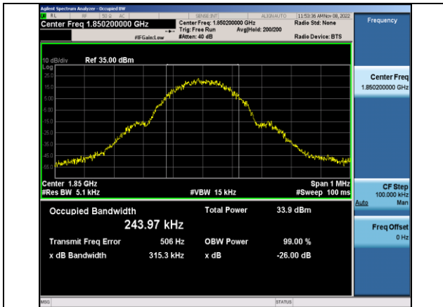
GPRS1900-512-0-0.3153
