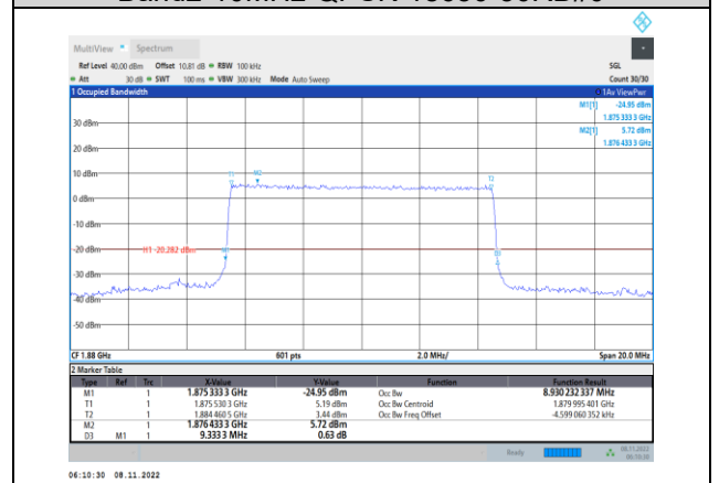
Band2-10MHz-QPSK-18900-50RB#0
