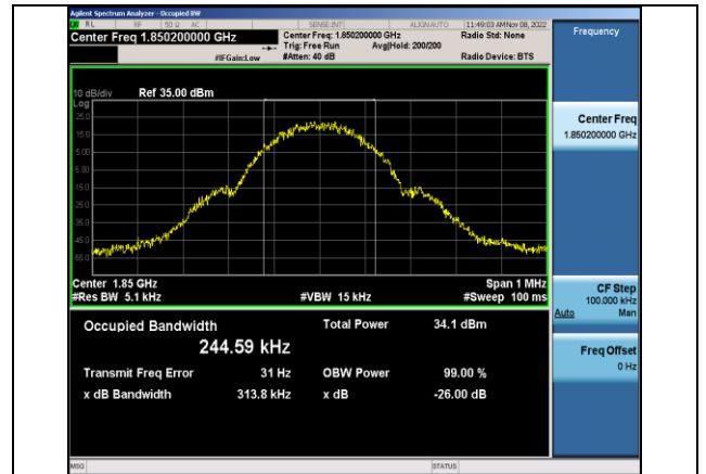
GSM1900-512-0-0.3138
