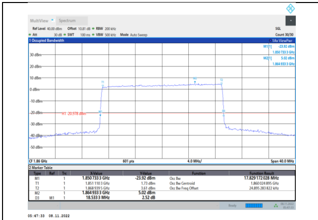
Band2-20MHz-16QAM-18700-100RB#0
