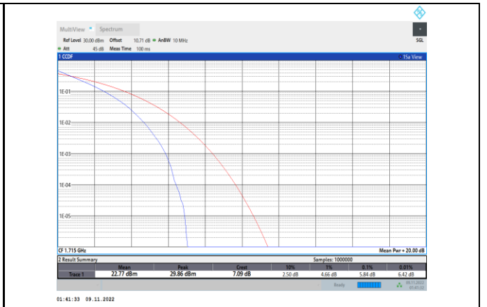
Band4-10MHz-QPSK-20000-50RB#0
