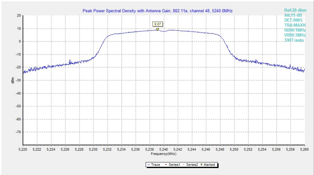
802.11a 6Mbps ch48 5240MHz
