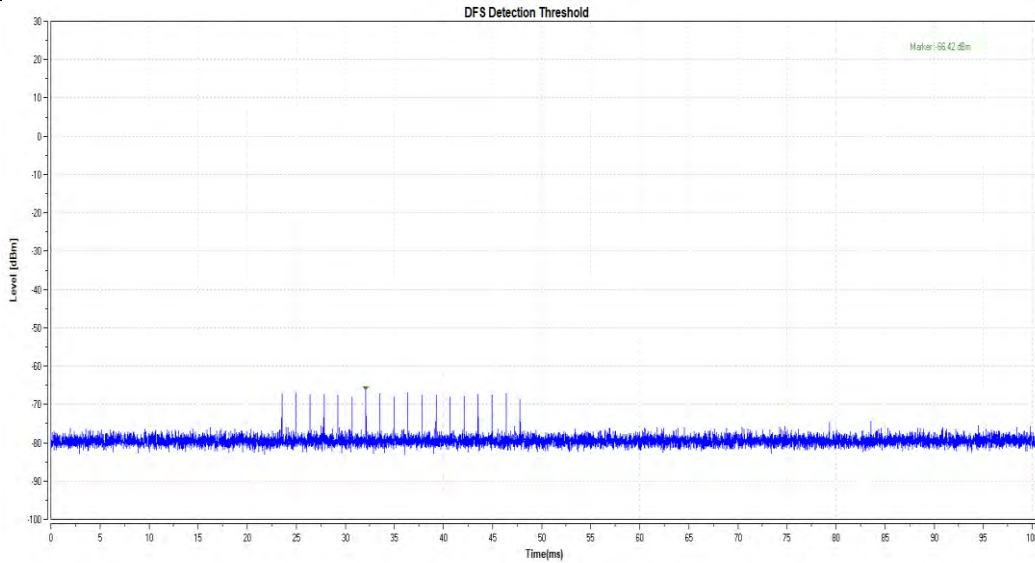
11AC80SISO_5530_Type0
