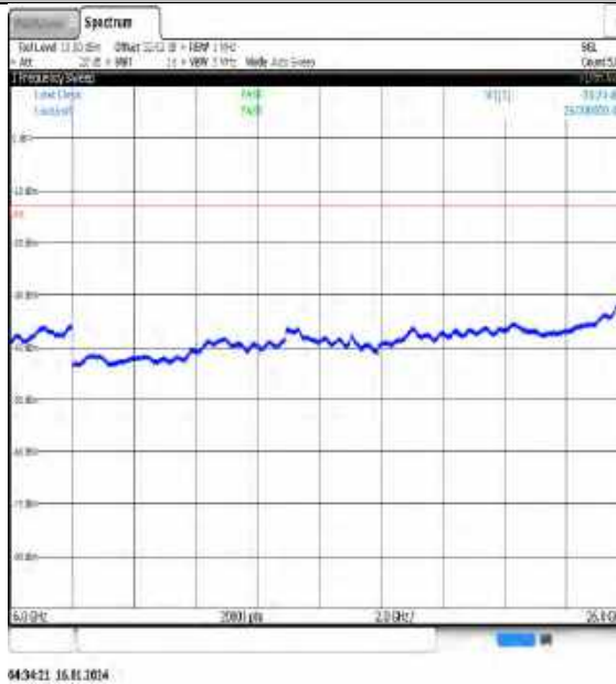
NTNV_N77-3450- 3550_PC3_30_90_M_TID2_NS_01_6000_26000_# #1
