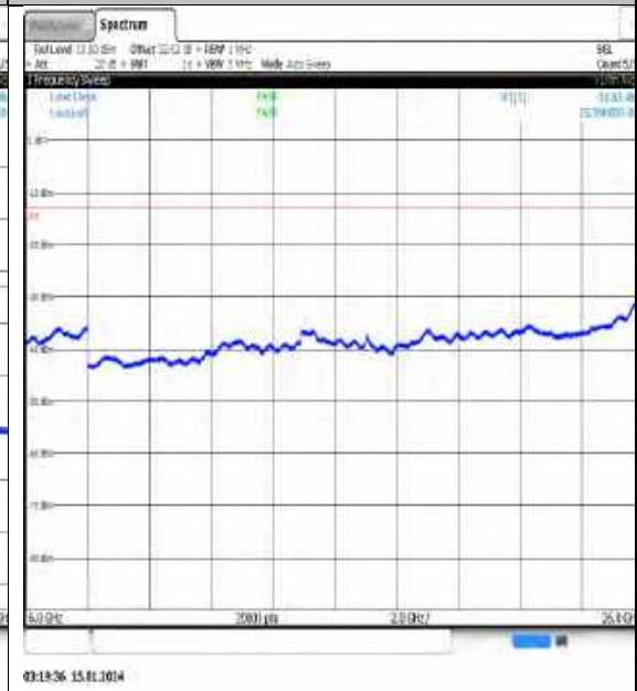
NTNV_N77-3450-3550_PC3_30_20_L_TID5_NS_01_6000_26000_#1
