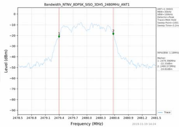
8DPSK_2480MHz_3DH5_SISO_ANT1
