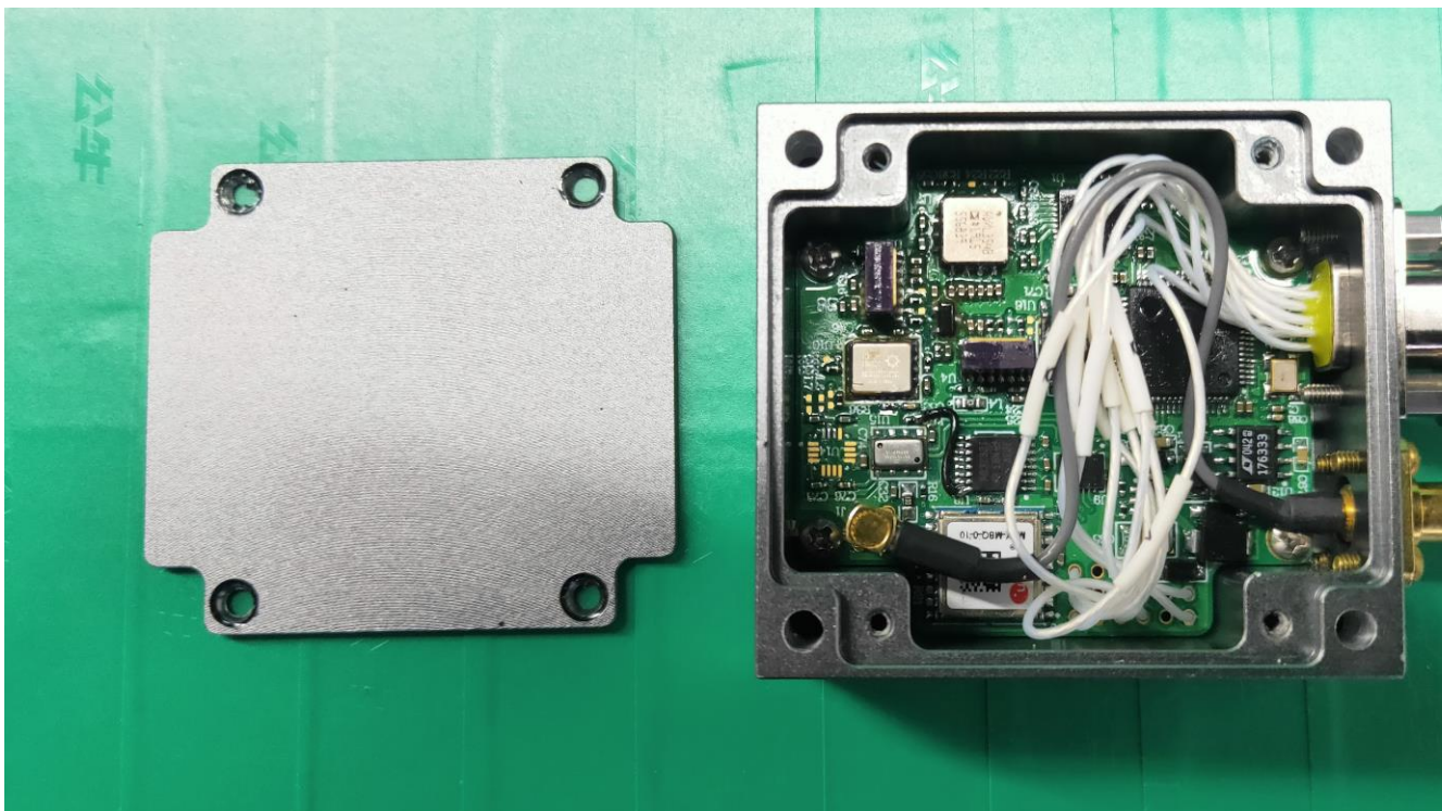
(18) EUT Photo
