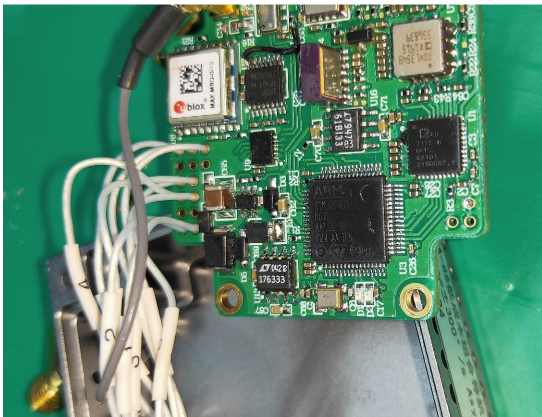
(24) EUT Photo
