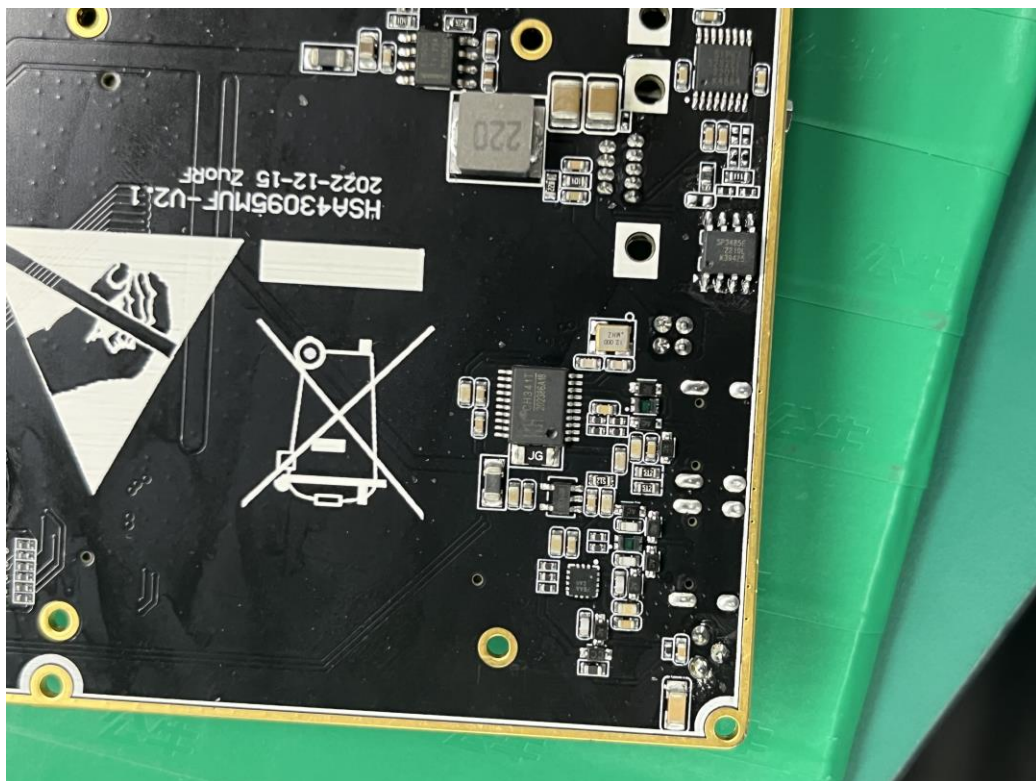
(14) EUT Photo
