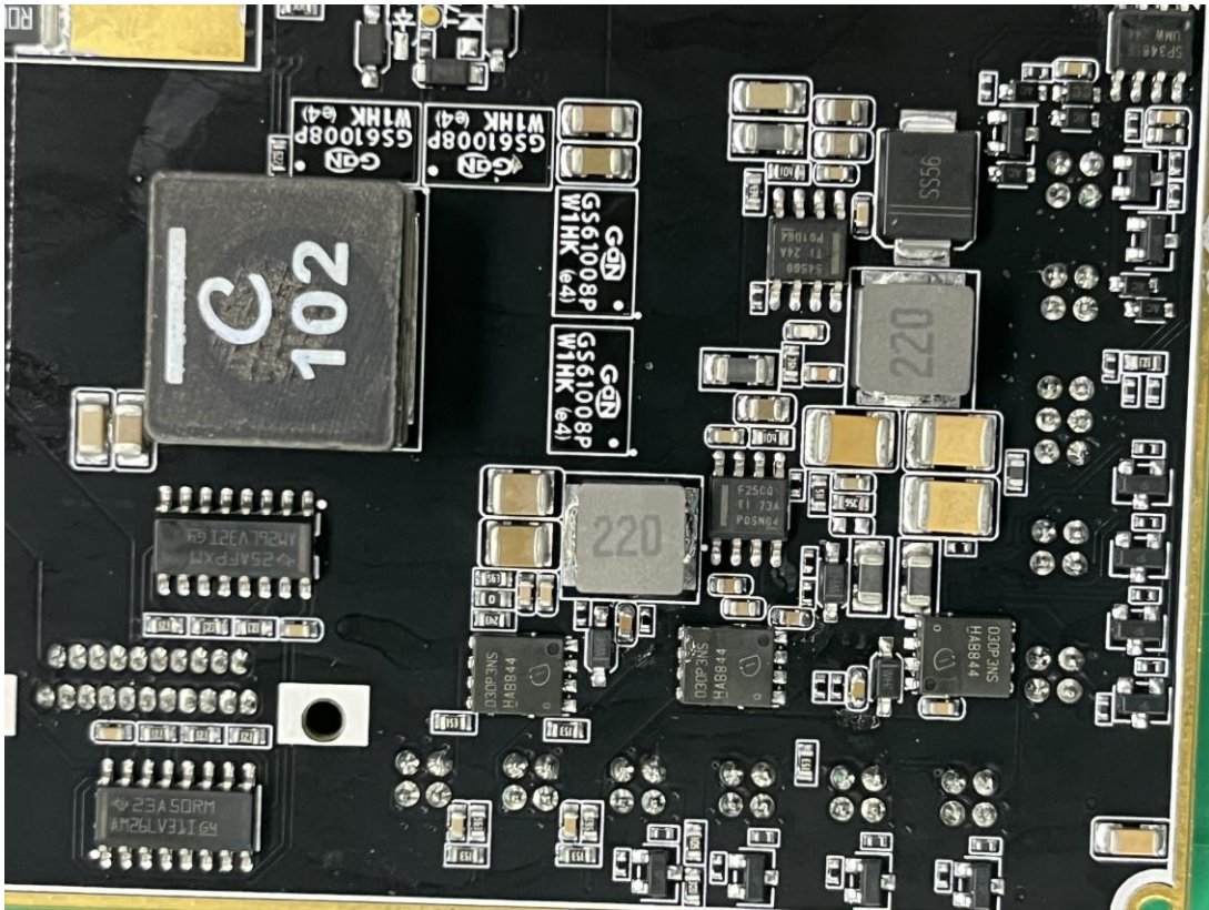
(12) EUT Photo
