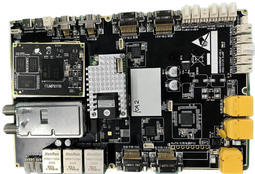
(2) EUT Photo
