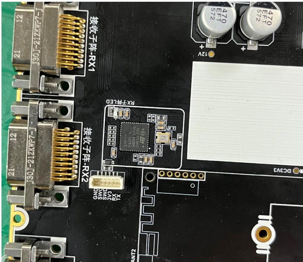
(10) EUT Photo
