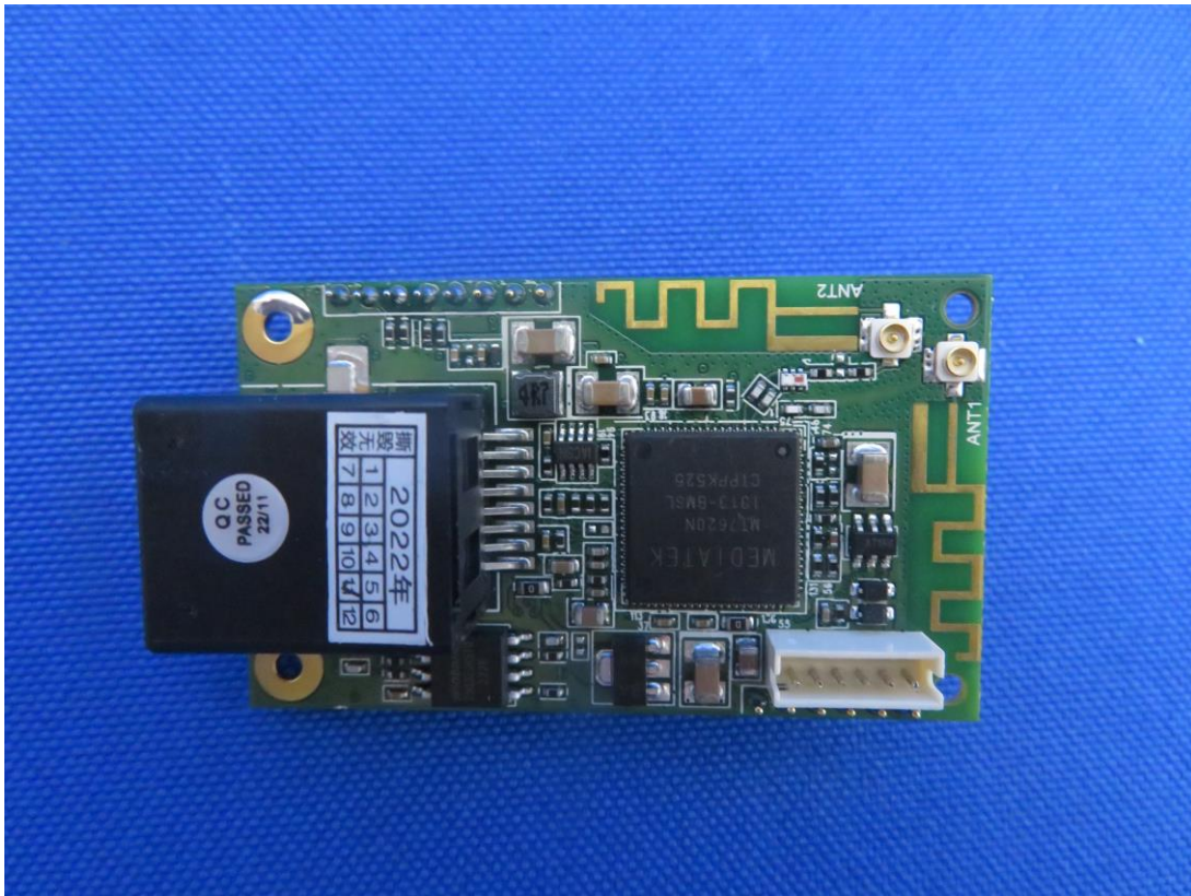
(16) EUT Photo
