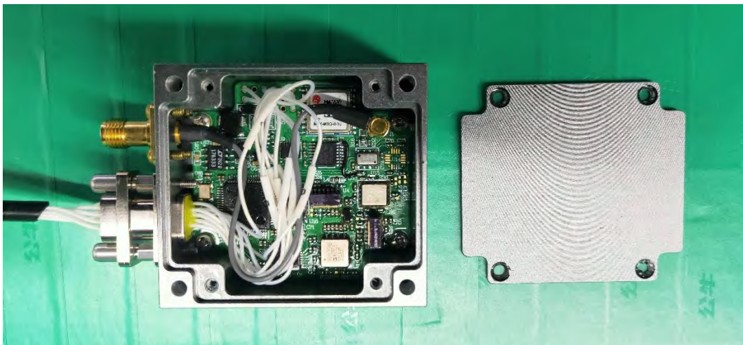
(40) EUT Photo
