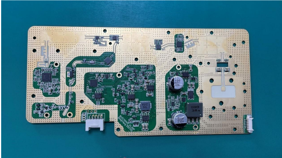
(9) EUT Photo
