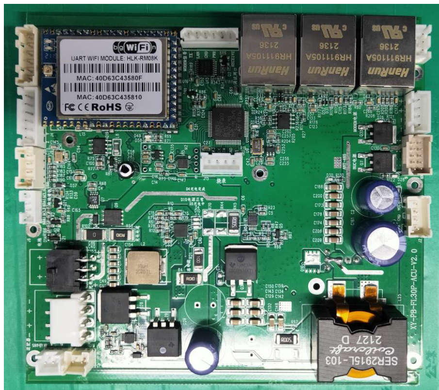
(6) EUT Photo
