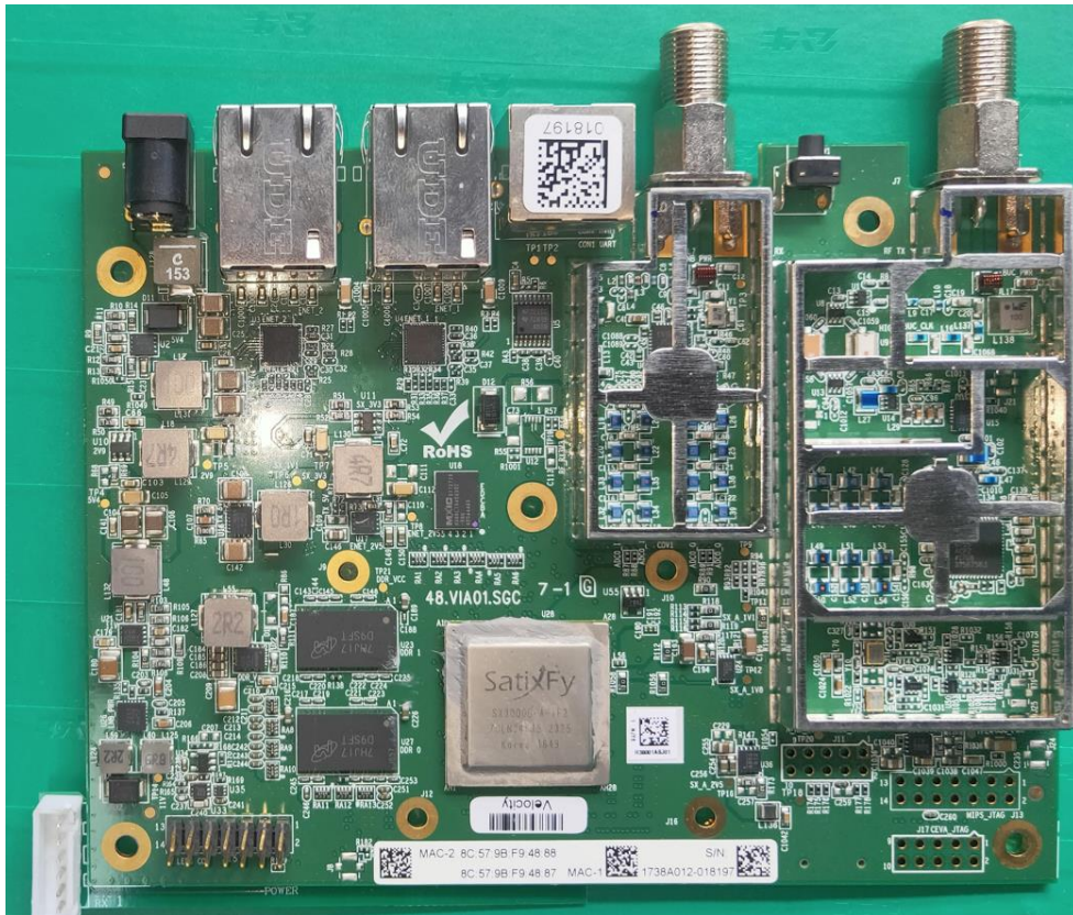
(6) EUT Photo
