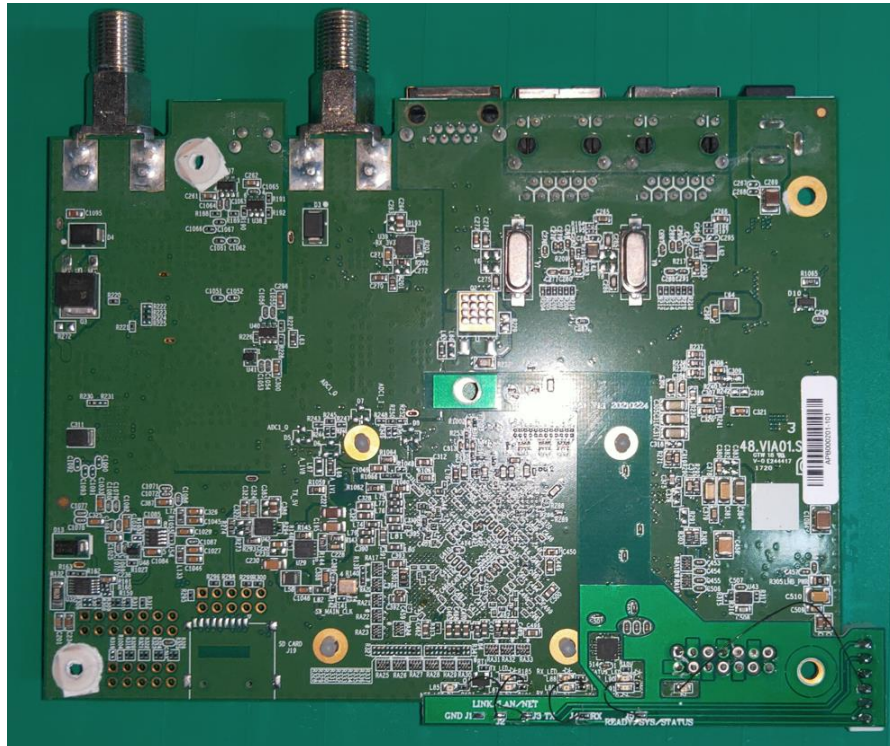
(3) EUT Photo
