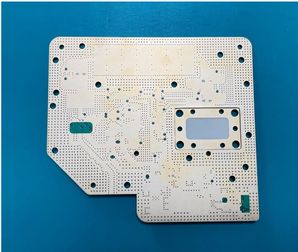
(10) EUT Photo
