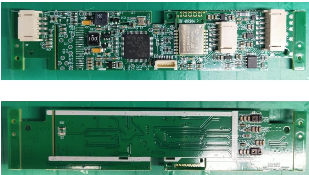
(14) EUT Photo
