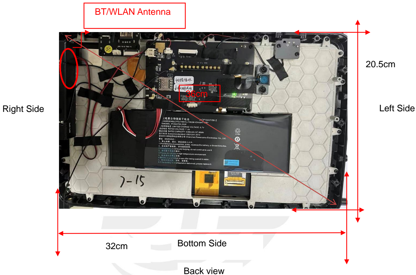
Top Side
