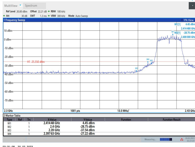
11G_Ant1_Low_2412
